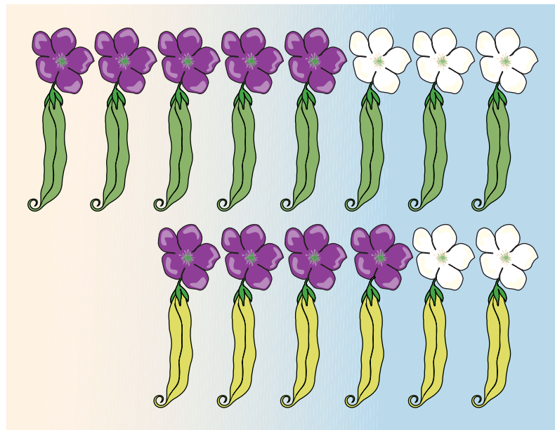
FIGURA 3-3 Chícharos usados en un estudio de genética
