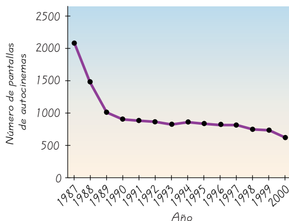
FIGURA 2-8 Datos de series de tiempo: número de pantallas de autocinemas
