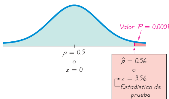
FIGURA 7-10 Método del valor P
