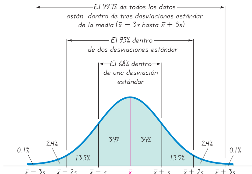
FIGURA 2-13 La regla empírica
