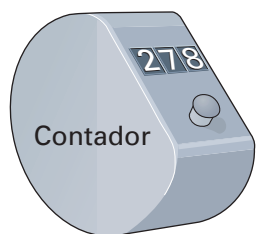
a) Variable aleatoria discreta: contador del número de asistentes a un cine.
