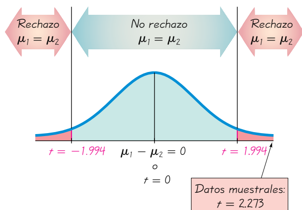
FIGURA 8-2 Distribución de valores \bar{x}_1 - \bar{x}_2
