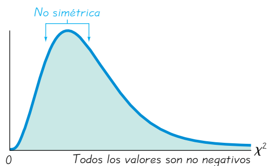
FIGURA 7-12 Propiedades de la distribución chi cuadrada
