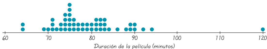
FIGURA 2-5 Gráfica de puntos de la duración de películas para niños
