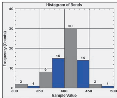
STATDISK
