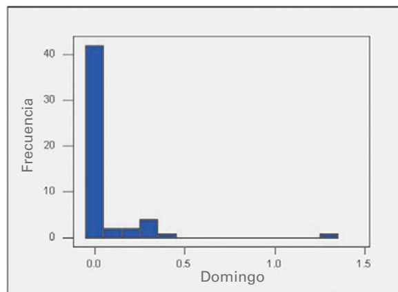
Minitab Histograma de las cantidades de lluvia de los domingos en Boston
