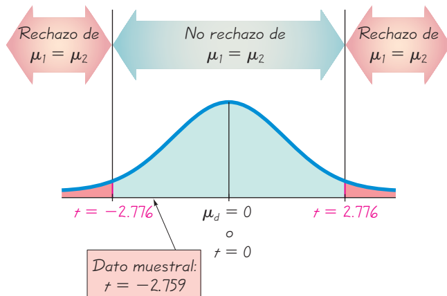
FIGURA 8-4 Distribución de diferencias d entre valores de datos apareados
