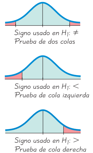
FIGURA 7-5 Pruebas de dos colas, cola izquierda, cola derecha
