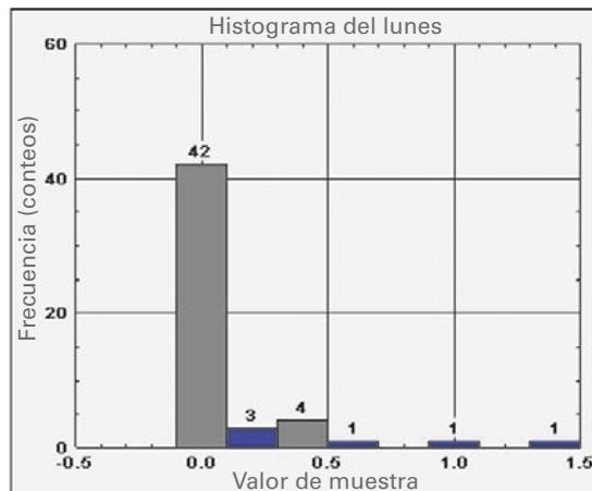
STATDISK
