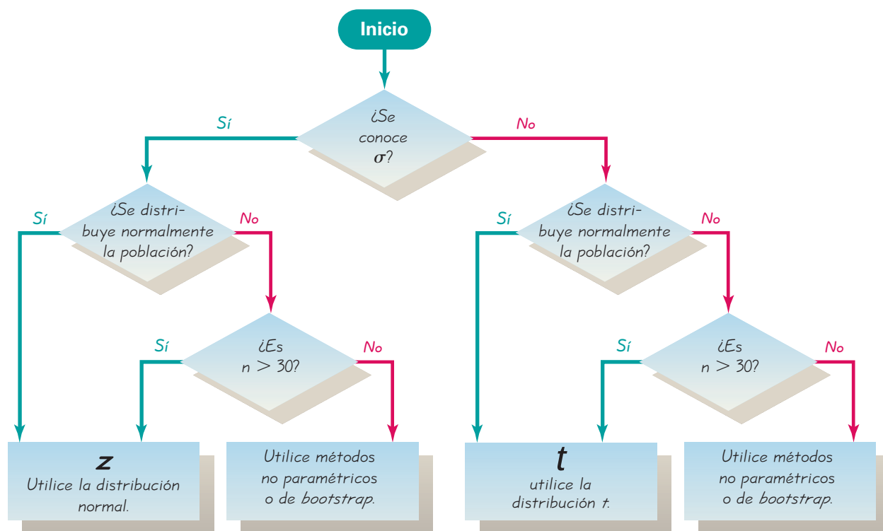
FIGURA 6-6 Elección entre z y t
