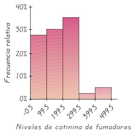
FIGURA 2-2 Histograma de frecuencias relativas
