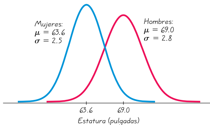
FIGURA 5-4 Estaturas de hombres y mujeres adultos
