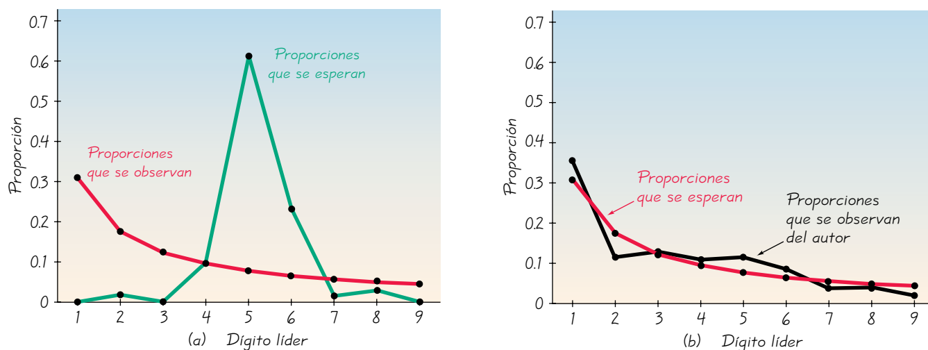
FIGURA 10-6 Comparación de las frecuencias que se observan y las frecuencias que se esperan con la ley de Benford
