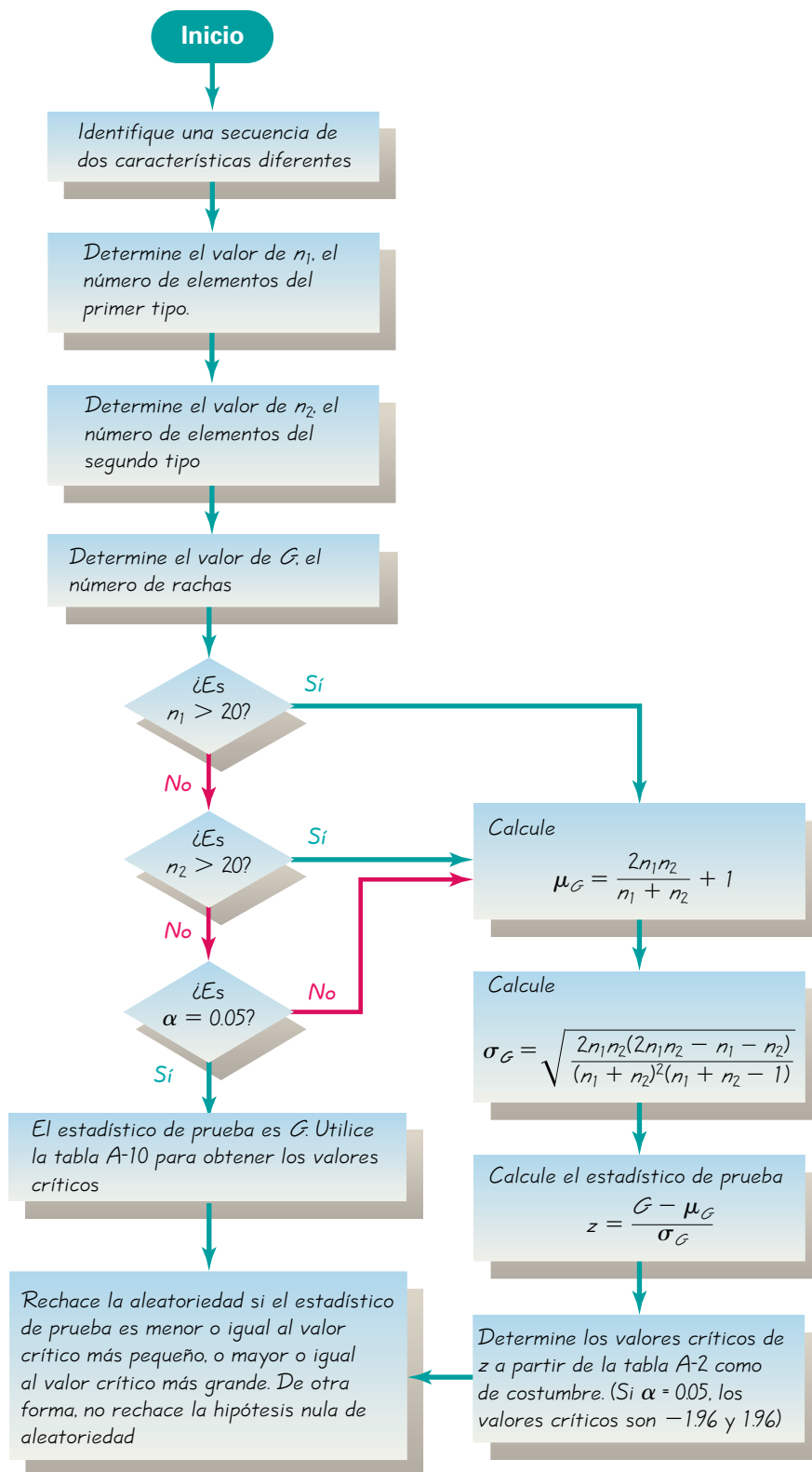
FIGURA 12-5 Prueba de rachas para detectar aleatoriedad
