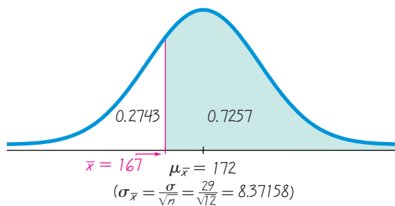
FIGURA 5-21(b) Medias de muestras de los pesos de 12 hombres
