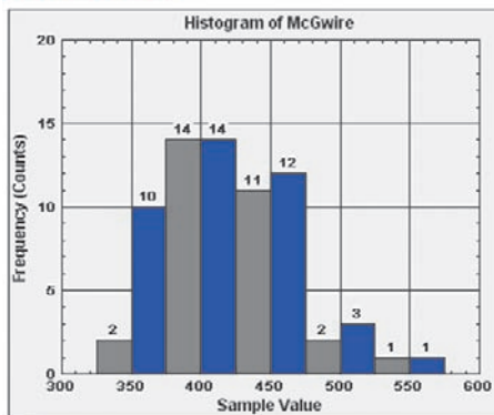
STATDISK
