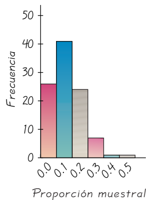
FIGURA 5-17 100 proporciones muestrales con n = 10 en cada muestra
