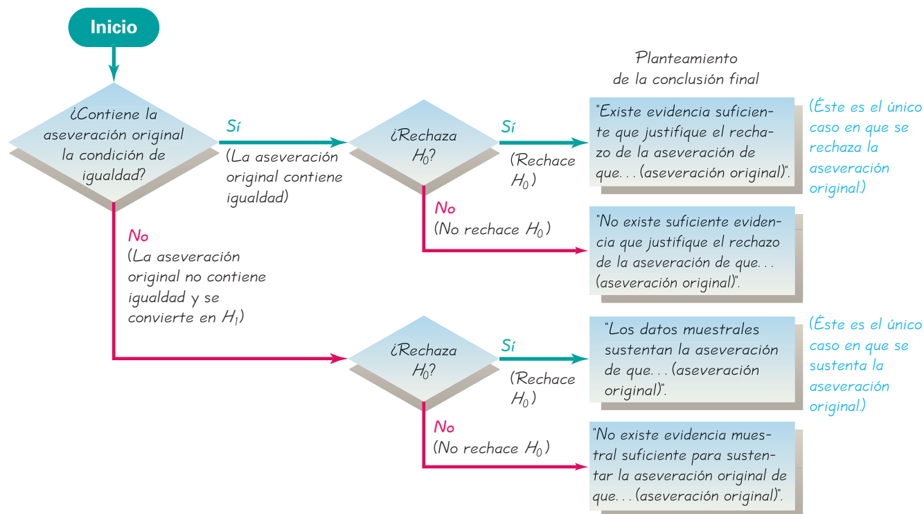
FIGURA 7-7 Conclusión final
