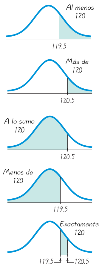
FIGURA 5-25 Uso de las correcciones por continuidad
