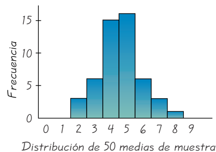
FIGURA 5-20 Distribución de 50 medias de muestra
