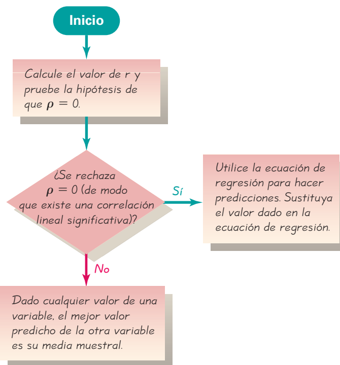
FIGURA 9-8 Procedimiento para hacer predicciones
