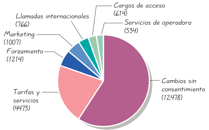
FIGURA 2-7 Gráfica circular de quejas en contra de las compañías telefónicas
