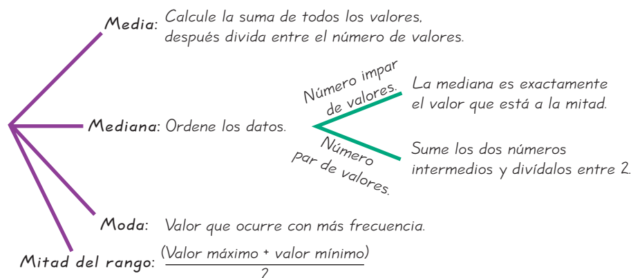
FIGURA 2-10 Procedimientos para calcular las medidas de tendencia central
