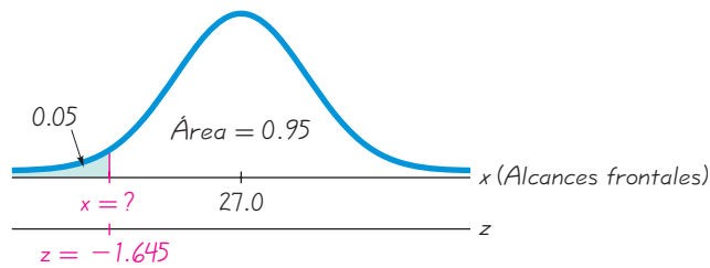
FIGURA 5-16 Cálculo del valor que separa al 95% superior
