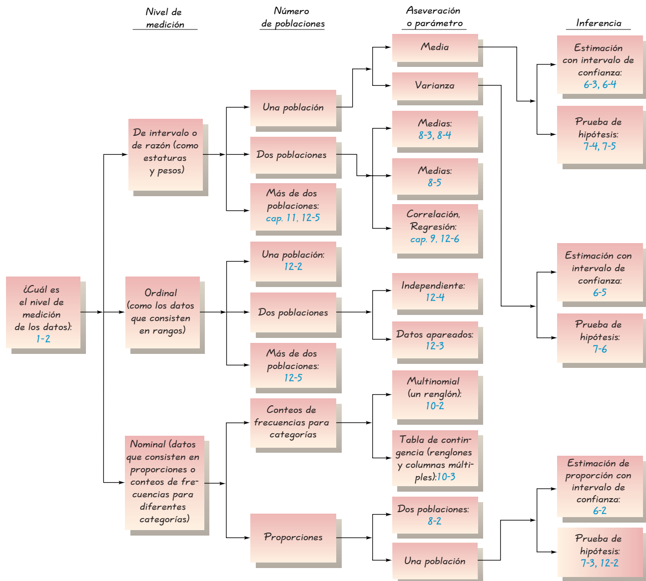
FIGURA 14-1 Selección del procedimiento adecuado
