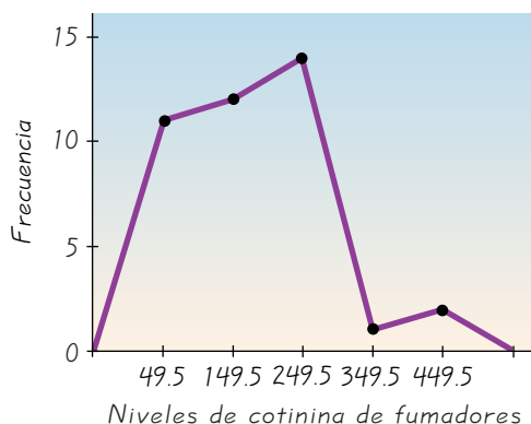
FIGURA 2-3 Polígono de frecuencias
