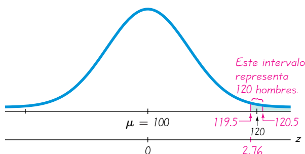
FIGURA 5-24 Búsqueda de la probabilidad de “al menos” 120 hombres entre 200 pasajeros
