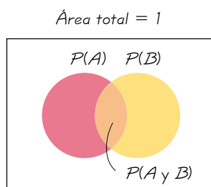
FIGURA 3-4 Diagrama de Venn que muestra sucesos traslapados
