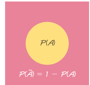
FIGURA 3-7 Diagrama de Venn para el complemento del suceso A
