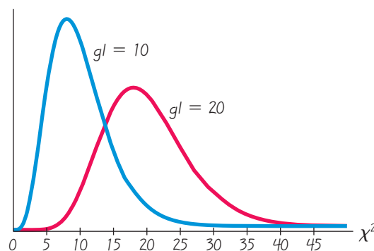
FIGURA 7-13 Distribución chi cuadrada para 10 y 20 grados de libertad
