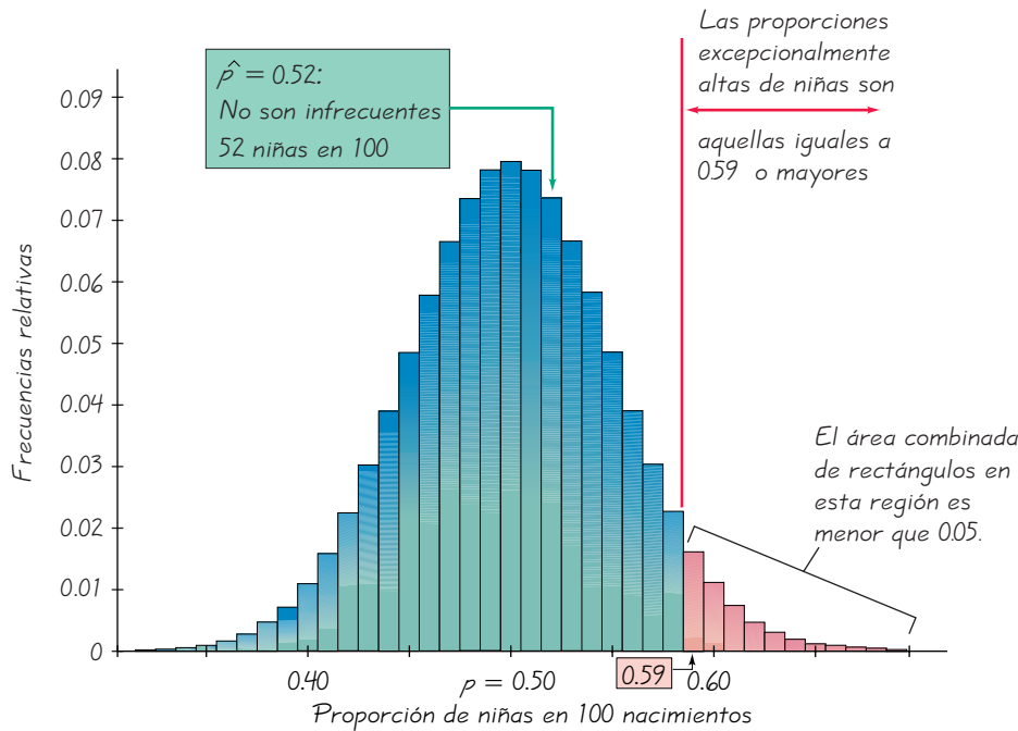
FIGURA 7-1 Distribución muestral de proporciones de niñas en 100 nacimientos
