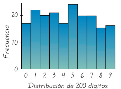
FIGURA 5-19 Distribución de 200 dígitos de los números del seguro social
