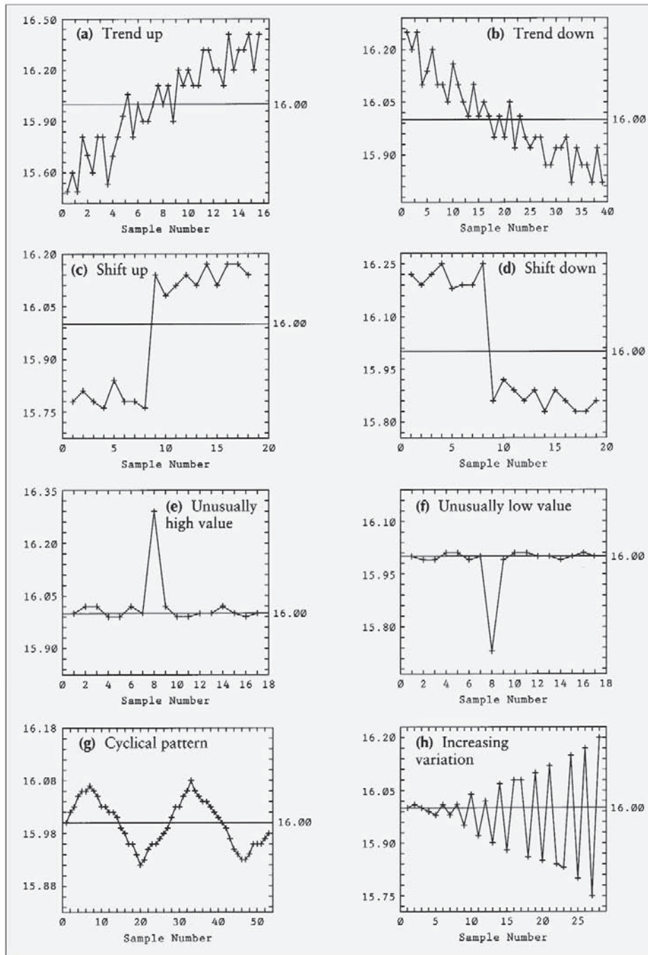
FIGURA 13-2 Procesos que no son estadísticamente estables
