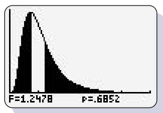
TI-83 Plus
