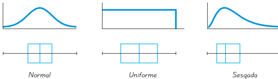
FIGURA 2-17 Gráficas de cuadro que corresponden a distribuciones normales, uniformes y sesgadas
