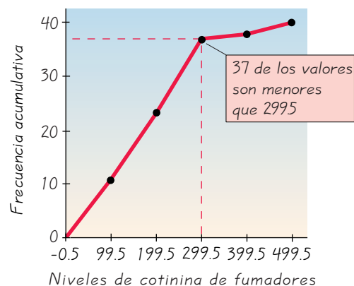
FIGURA 2-4 Ojiva
