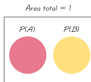
FIGURA 3-5 Diagrama de Venn que muestra sucesos no traslapados
