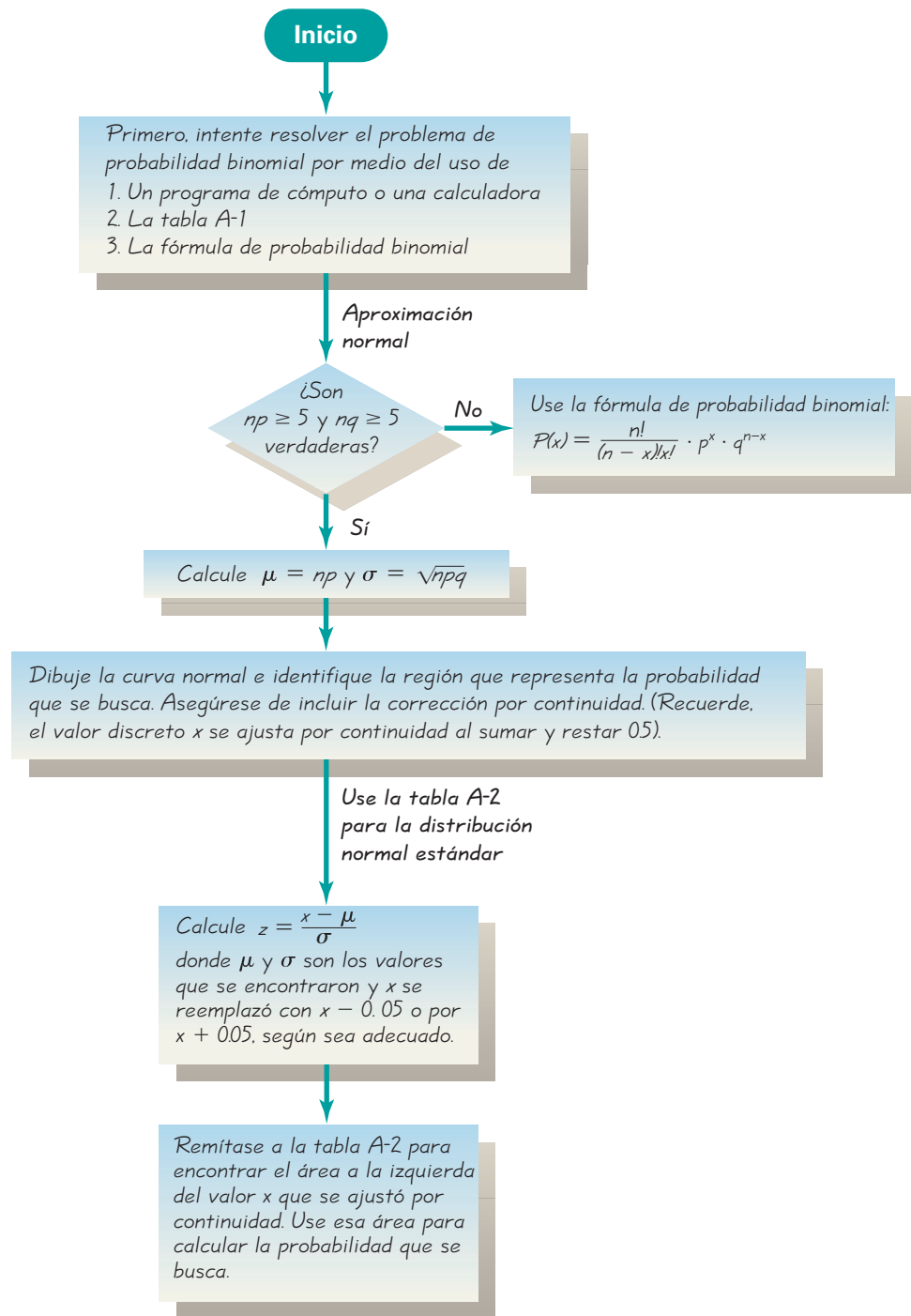
FIGURA 5-23 Uso de la distribución normal como aproximación de la distribución binomial
