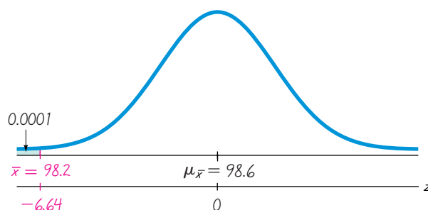
FIGURA 5-22 Distribución de temperaturas corporales medias, para muestras de tamaño n = 106
