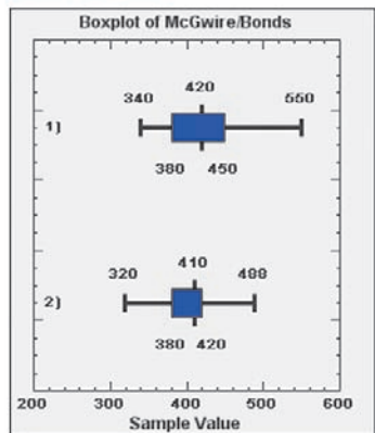
STATDISK
