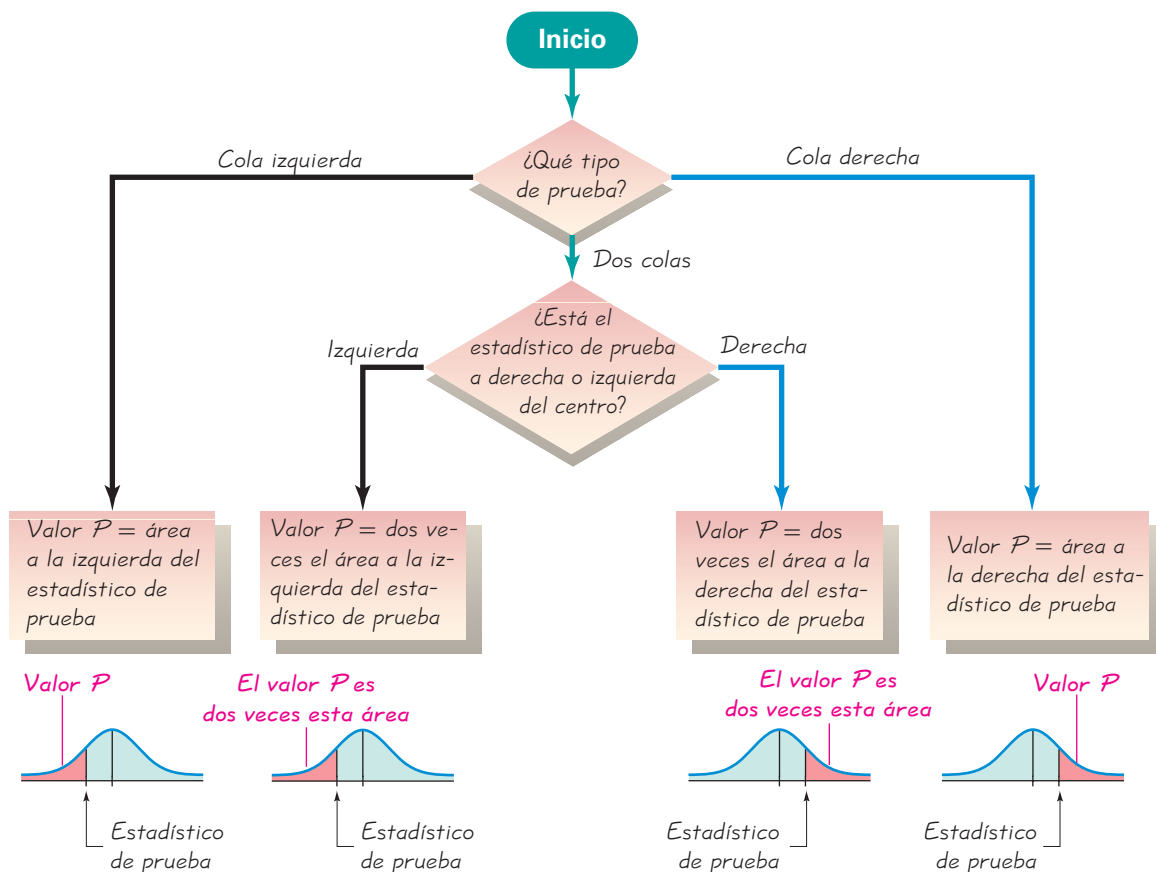
FIGURA 7-6 Procedimiento para el cálculo de los valores P
