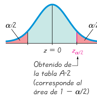
FIGURA 6-2 Valor crítico z_{\alpha/2} en la distribución normal estándar
