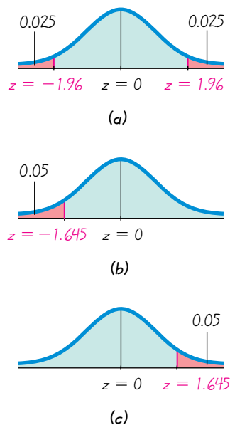
FIGURA 7-4 Cálculo de valores críticos
