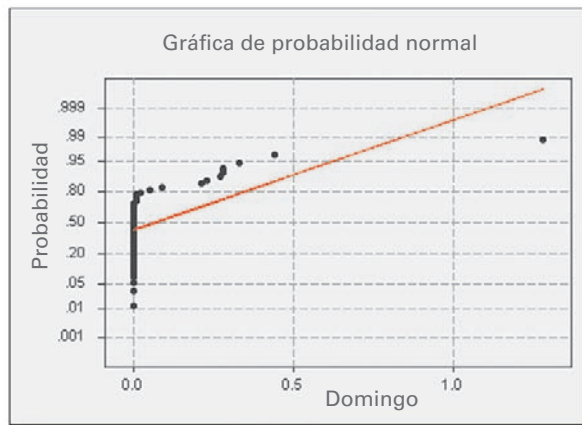
Minitab Gráfica de probabilidad normal de las cantidades de lluvia de los domingos en Boston
