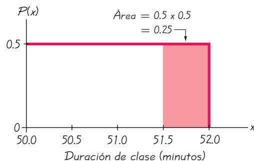
FIGURA 5-3 Uso del área para el cálculo de la probabilidad
