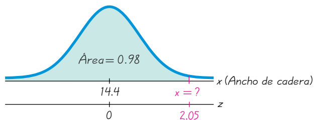
FIGURA 5-15 Distribución del ancho de cadera de hombres
