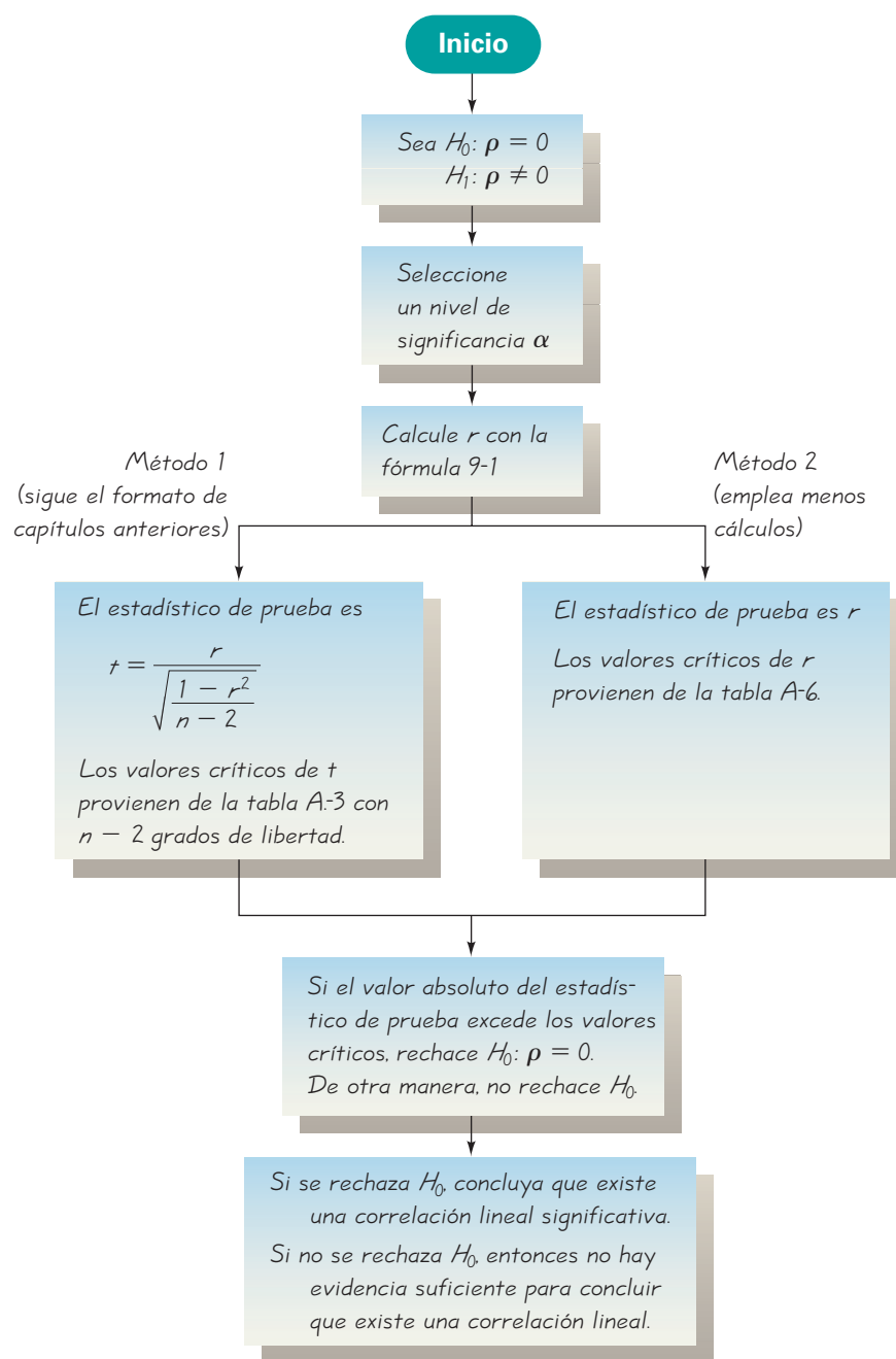
FIGURA 9-4 Prueba de hipótesis para una correlación lineal
