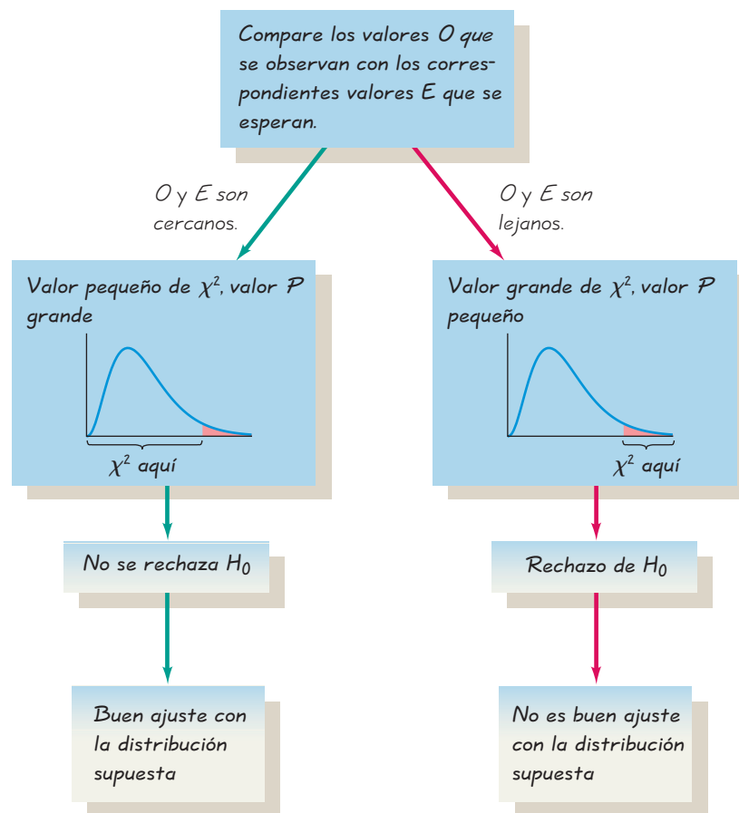
FIGURA 10-3 Relaciones entre el estadístico de prueba \chi^2 , el valor P y la bondad de ajuste
