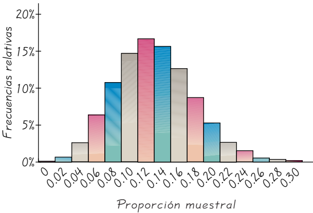
FIGURA 5-18 10,000 proporciones muestrales con n = 50 en cada muestra
