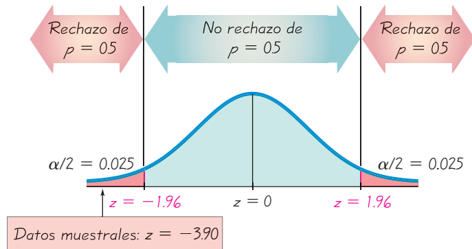
FIGURA 12-2 Prueba de la aseveración de prácticas de contratación injustas
