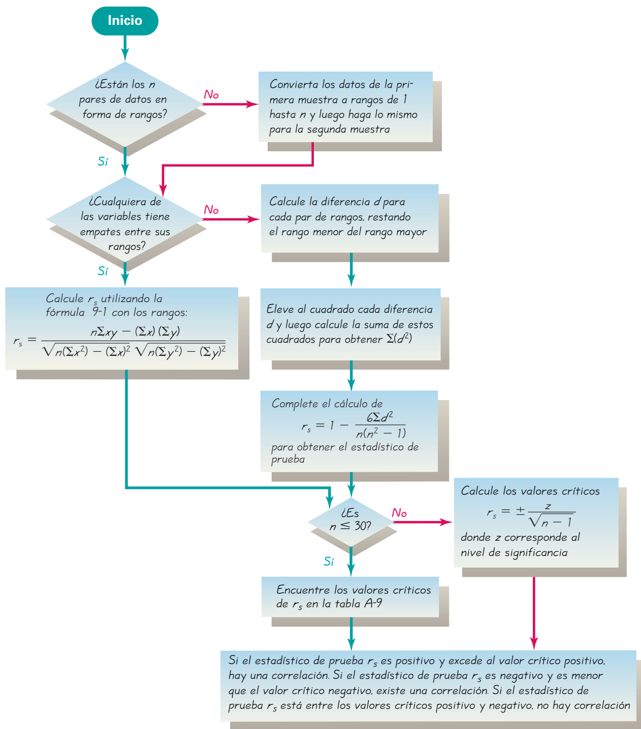
FIGURA 12-4 Procedimiento de correlación de rangos para probar H_0: \rho_s = 0
