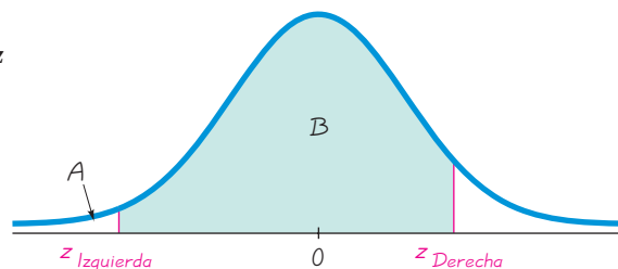
FIGURA 5-9 Cálculo del área entre dos puntuaciones z
