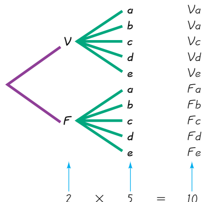
FIGURA 3-8 Diagrama de árbol de reactivos de examen
