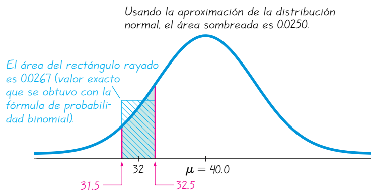
FIGURA 5-26 Uso de la corrección por continuidad de la audiencia televisiva
