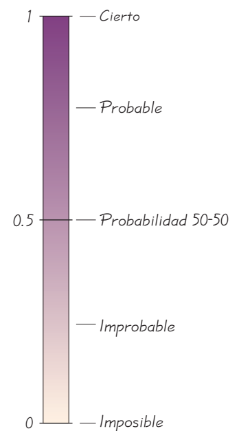
FIGURA 3-2 Valores posibles para probabilidades
