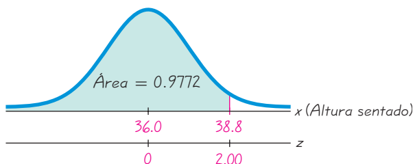
FIGURA 5-13 Distribución normal de la altura de hombres sentados
