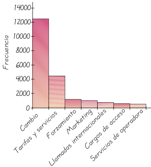
FIGURA 2-6 Gráfica de Pareto de quejas en contra de las compañías telefónicas
