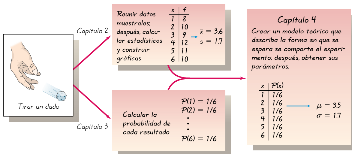
FIGURA 4-1 Combinación de métodos descriptivos y probabilidades para formar un modelo teórico de comportamiento
