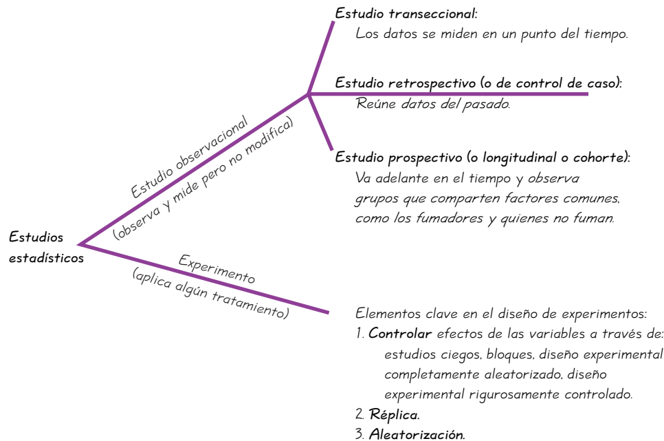
FIGURA 1-3 Elementos de los estudios estadísticos
