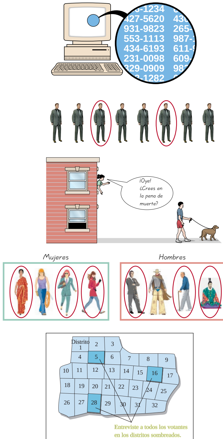
FIGURA 1-4 Métodos de muestreo comunes
