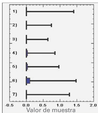
STATDISK
