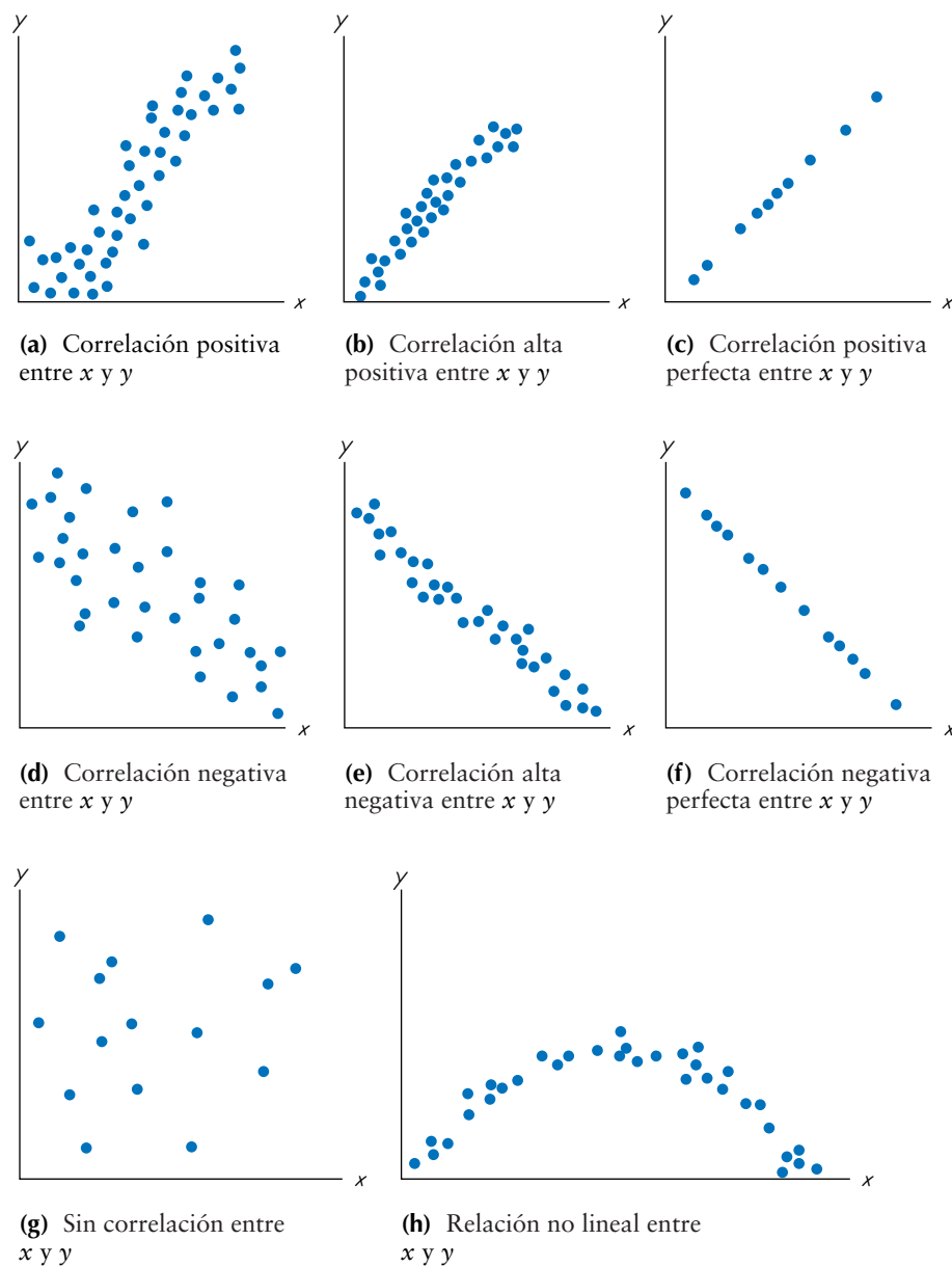
FIGURA 9-2 Diagramas de dispersión
