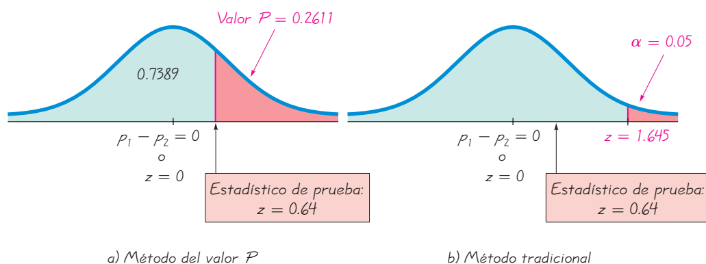
FIGURA 8-1
