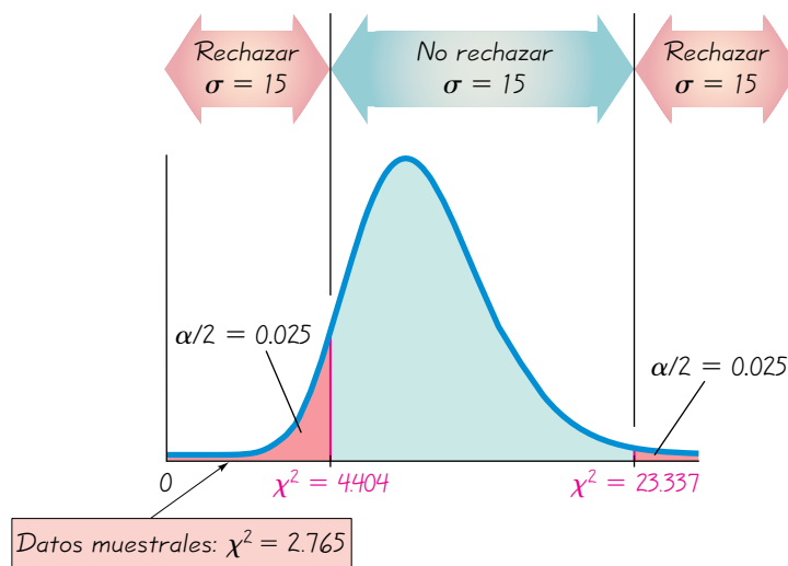
FIGURA 7-14 Prueba de la aseveración de que \sigma = 15
