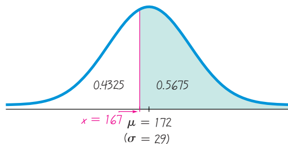
FIGURA 5-21(a) Distribución de pesos individuales de hombres
