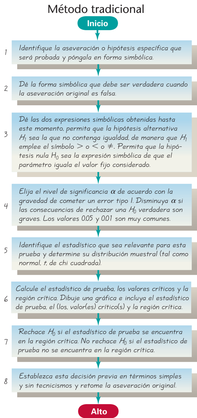
FIGURA 7-8 Método tradicional
