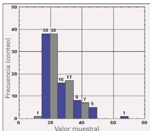
STATDISK
