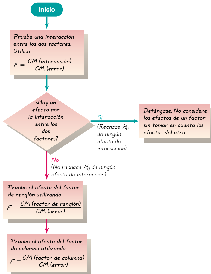
FIGURA 11-3 Procedimiento del ANOVA de dos factores
