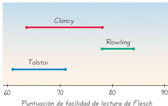
FIGURA 6-7 Comparación de intervalos de confianza
