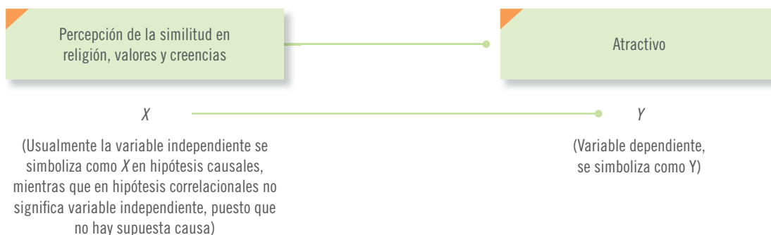
Figura 6.2 Esquema de relación causal bivariada.
