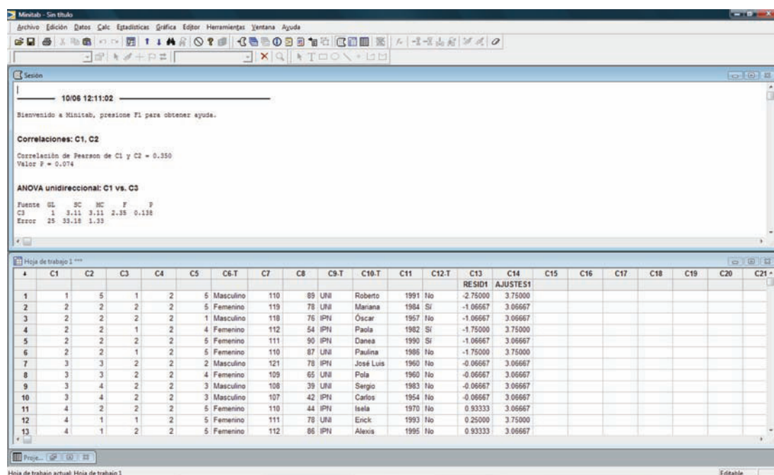
Figura 10.2 Pantalla de Minitab.
