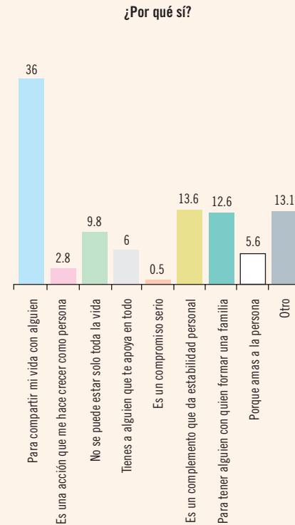
Figura 10.27 Razones del “sí”.
