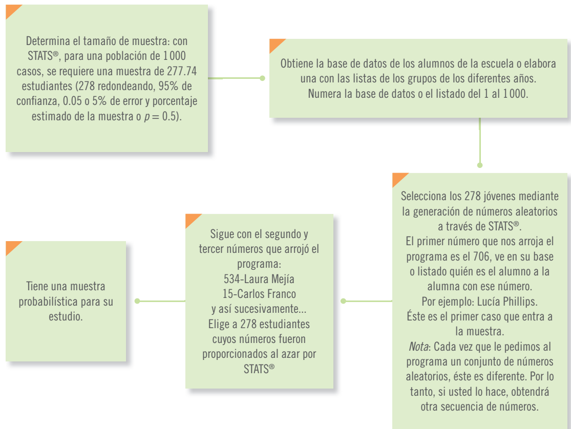
Figura 8.5 Ejemplo del procedimiento para elegir los casos de una muestra aleatoria simple usando STATS®.
