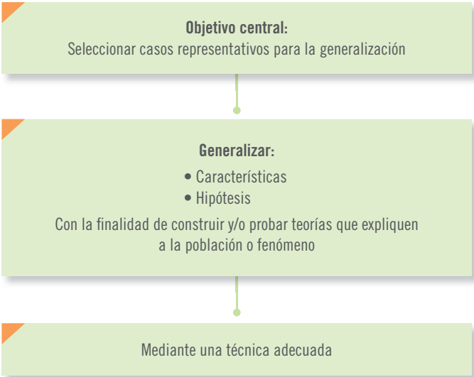
Figura 8.1 Esencia del muestreo cuantitativo.
