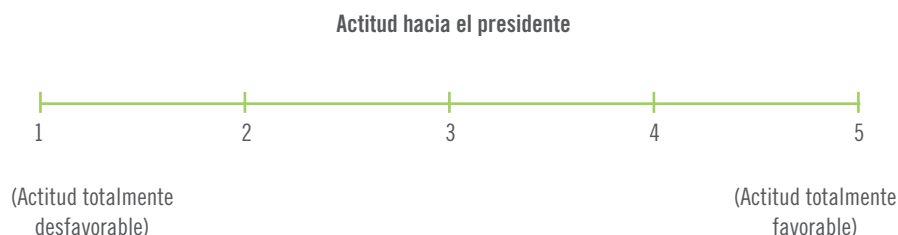
Figura 10.7 Ejemplo de escala con rango potencial.
