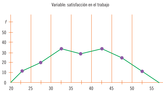
Figura 10.5 Ejemplo de un polígono de frecuencias.
