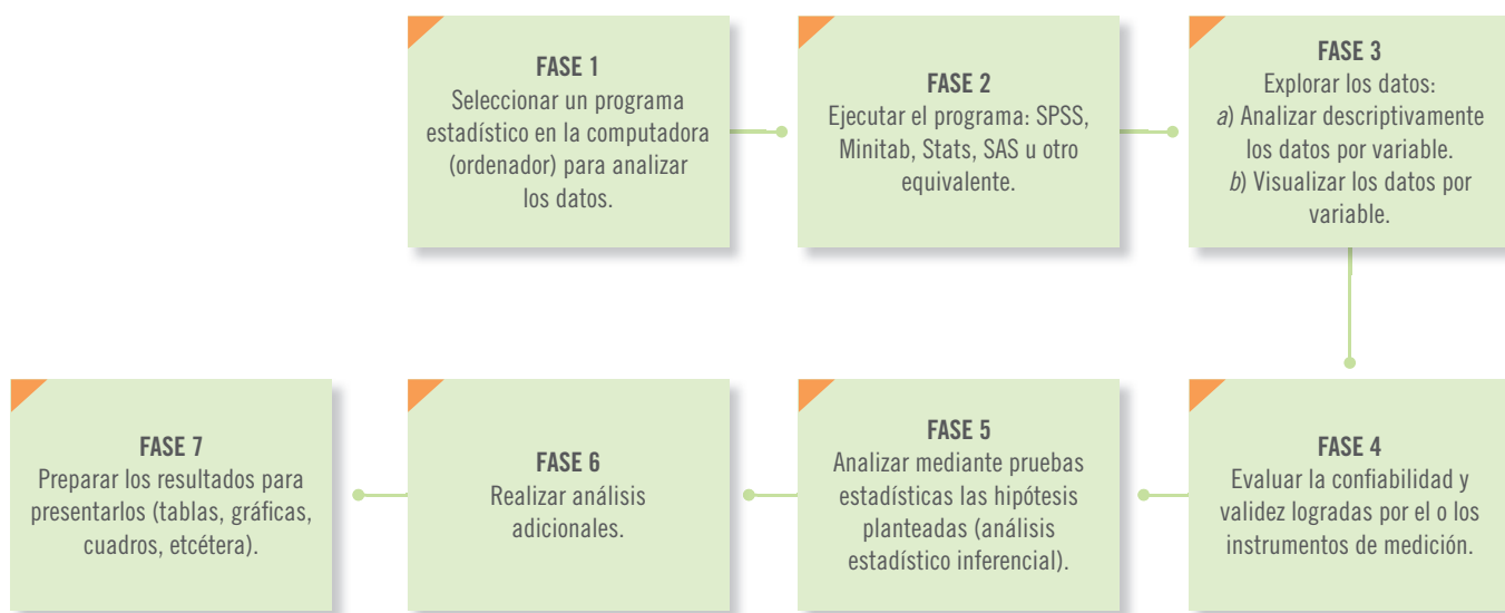
Figura 10.1 Proceso para efectuar análisis estadístico.
