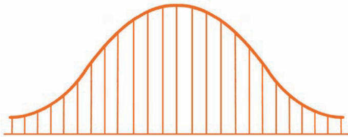
Figura 10.14 Distribución muestral de medias.
