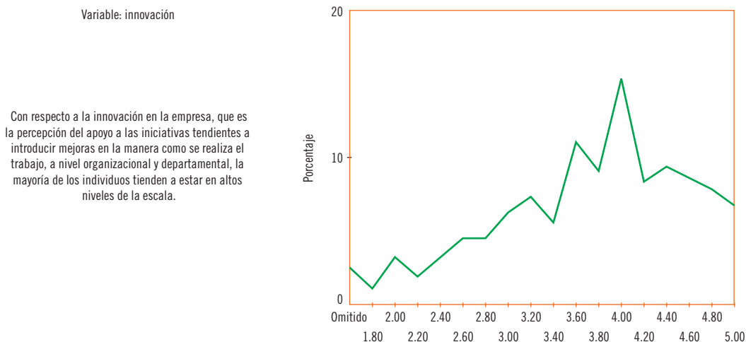
Figura 10.6 Ejemplo de un polígono de frecuencias con la variable innovación.
