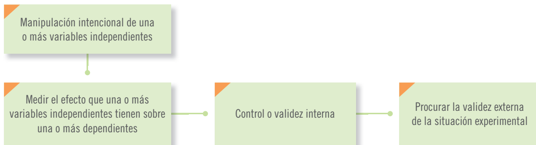
Figura 7.3 Requisitos de un experimento.
