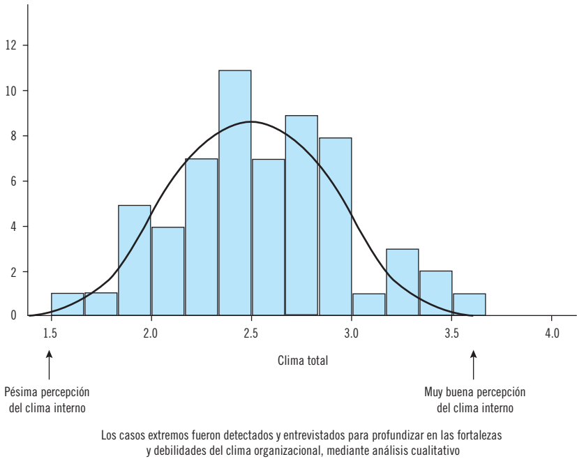
Figura 17.21 Análisis de casos extremos a partir de una distribución del clima organizacional en una empresa transportista.
