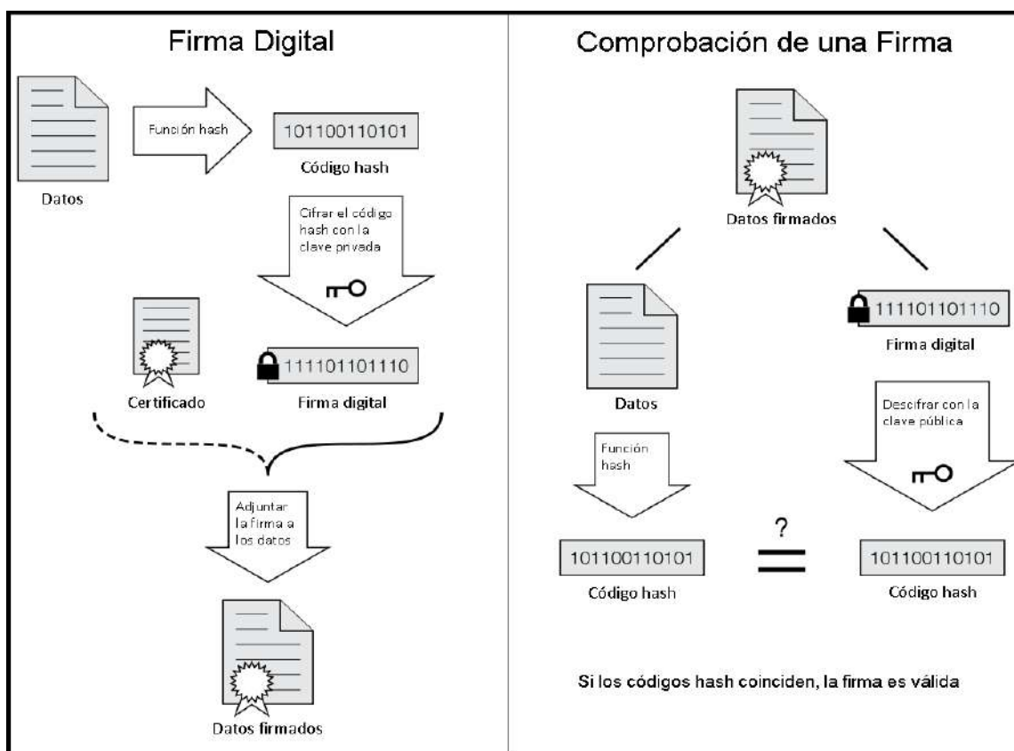
Figura 6.4 Funcionamiento de la Firma Digital. ( http://www.esacademic.com/ )
