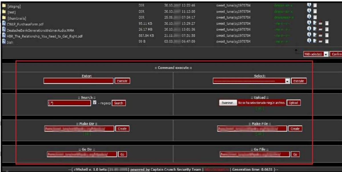
Figura 7.59 Opciones de la Shell – Web Analizada.
