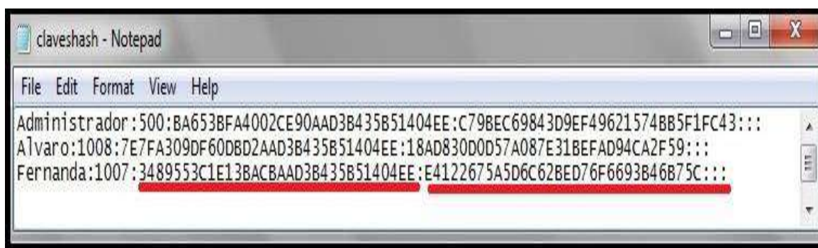
Figura 6.11 Archivo con los hashes obtenidos – Pwdump.
