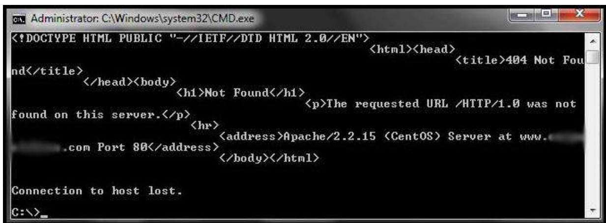
Figura 4.42.2 Resultado de una consulta telnet – D.O.S
