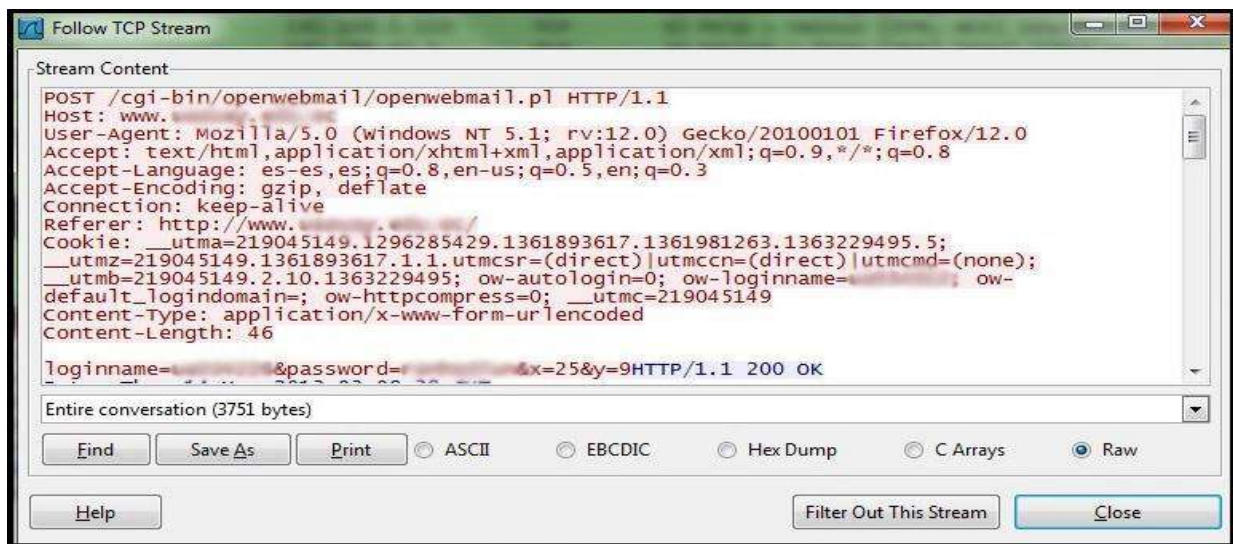
Figura 5.8 Visualización de un paquete con información de password - Wireshark.
