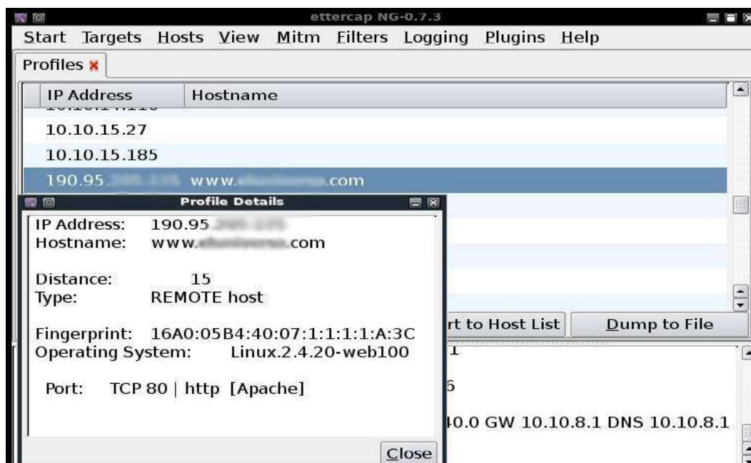
Figura 4.28 Escaneo Pasivo a un Sitio Web con Ettercap – Linux.
