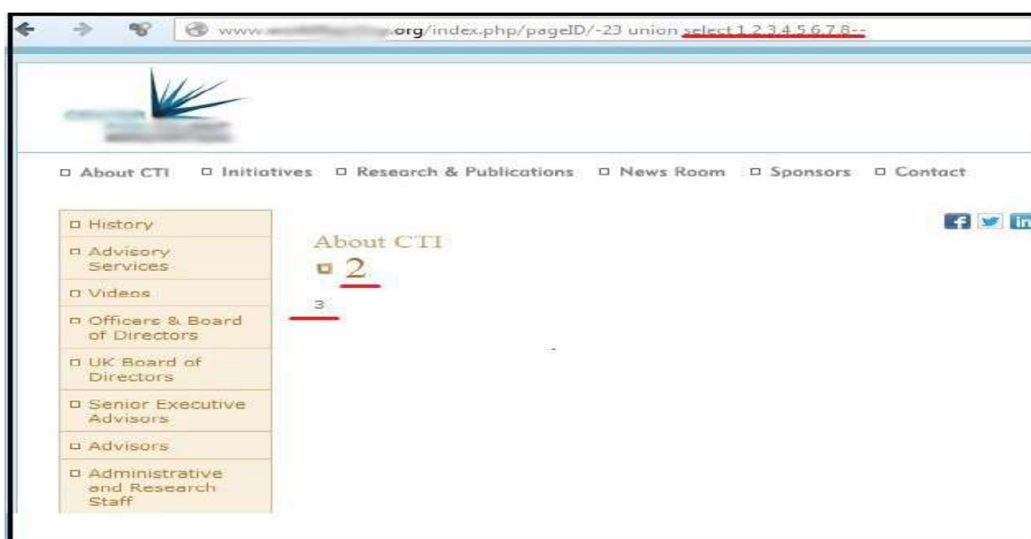
Figura 7.48 Visualización de los campos disponibles – Web Analizada.
