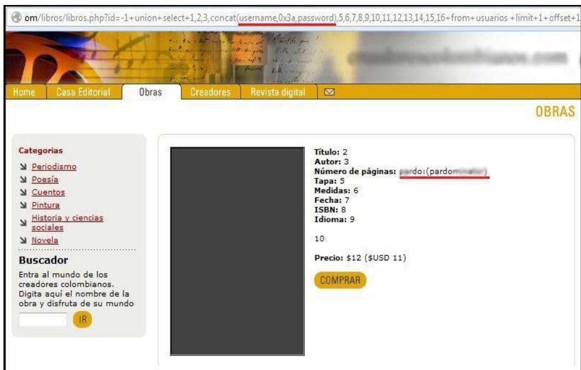
Figura 7.36 Consulta SQL para obtener usuarios y claves– Web Analizada.
