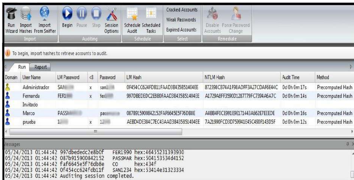
Figura 6.16 Resultado del ataque – L0phtCrack.
