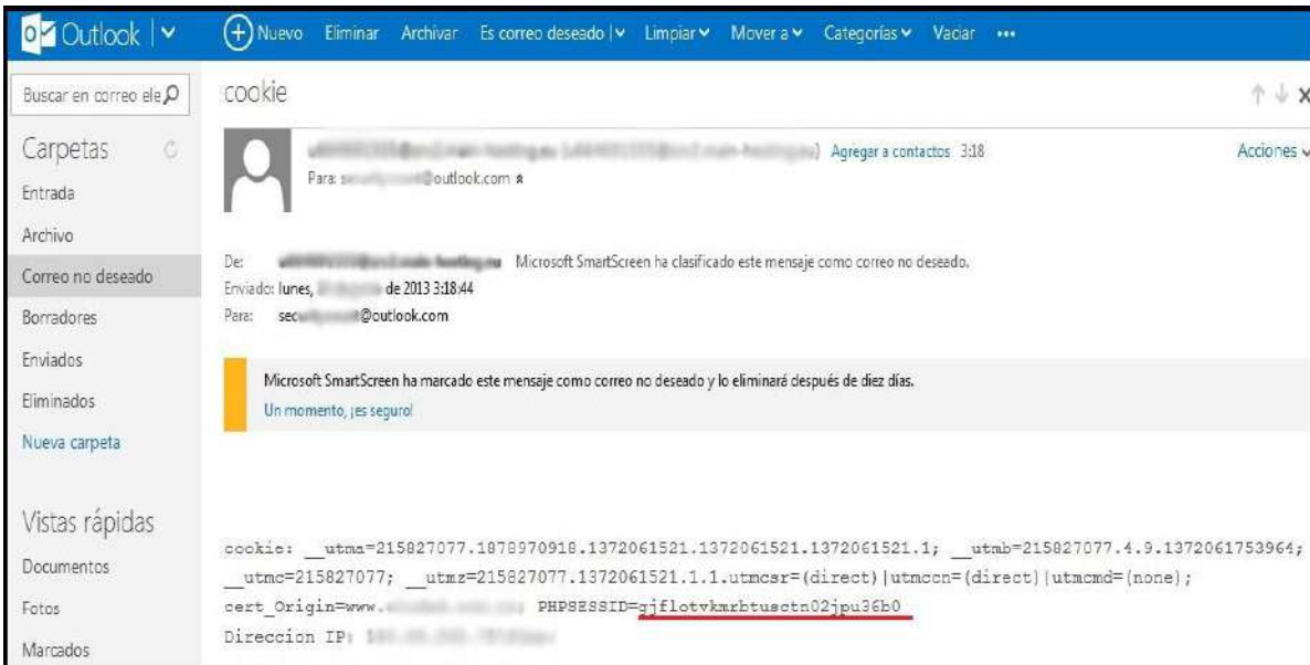
Figura 7.23 Correo recibido por el atacante.
