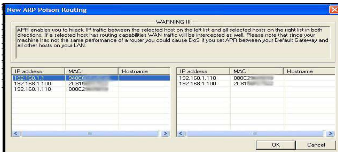
Figura 5.12 Selección de IPs para realizar una interceptación de tráfico – Cain y Abel.
