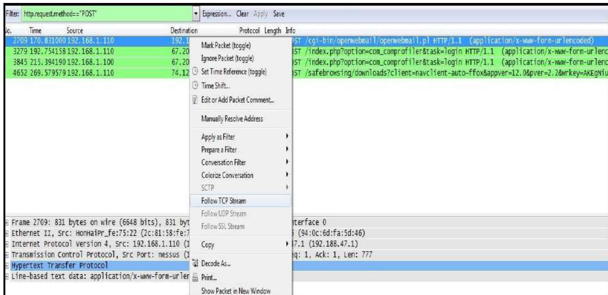
Figura 5.7 Sniffer a un equipo - Wireshark.
