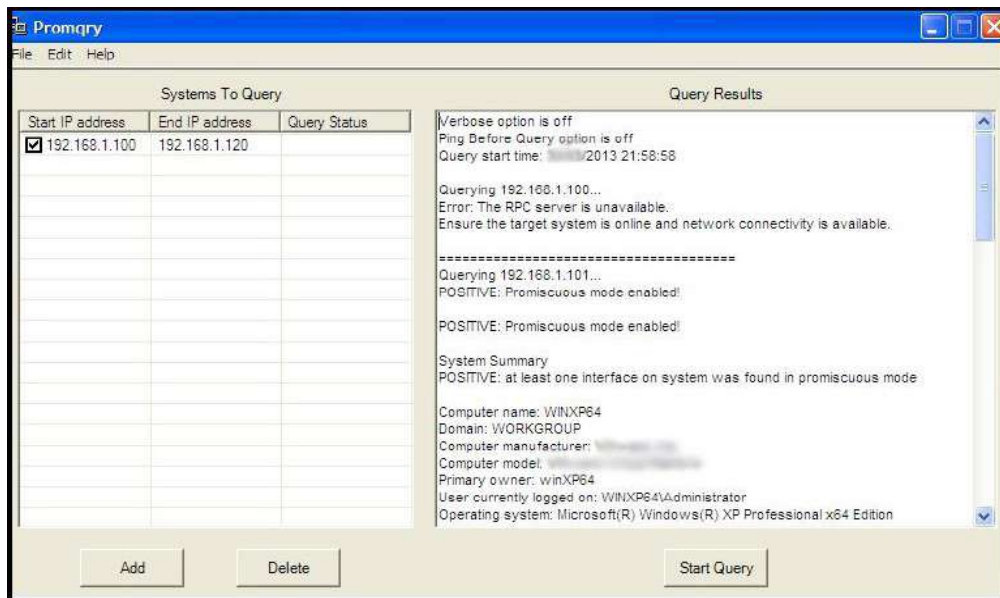
Figura 5.38 Ejecución de la herramienta Promqry – Windows.
