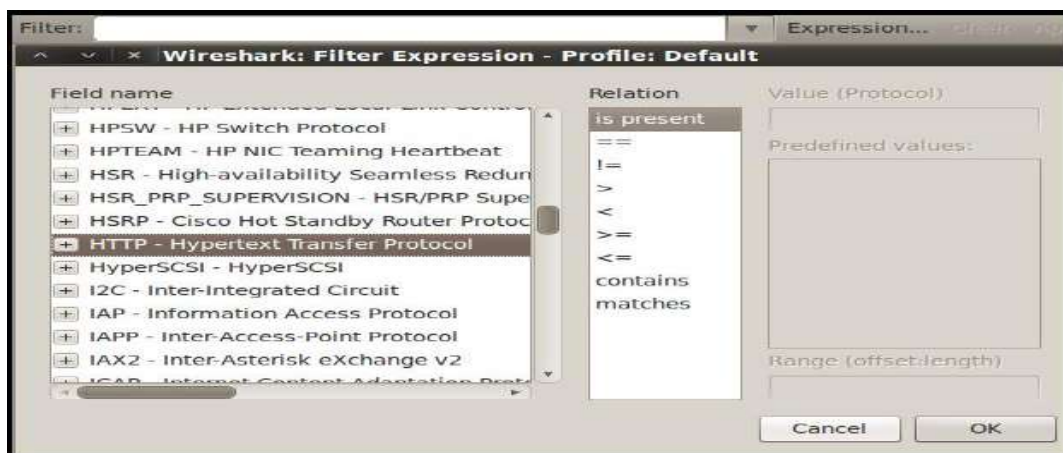
Figura 5.2 Barra y menú de Filtros de Wireshark.
