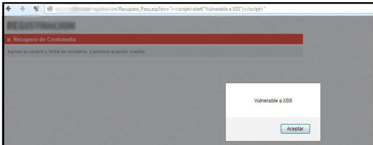
Figura 7.17 Testeo de vulnerabilidad XSS – Web Analizada.
