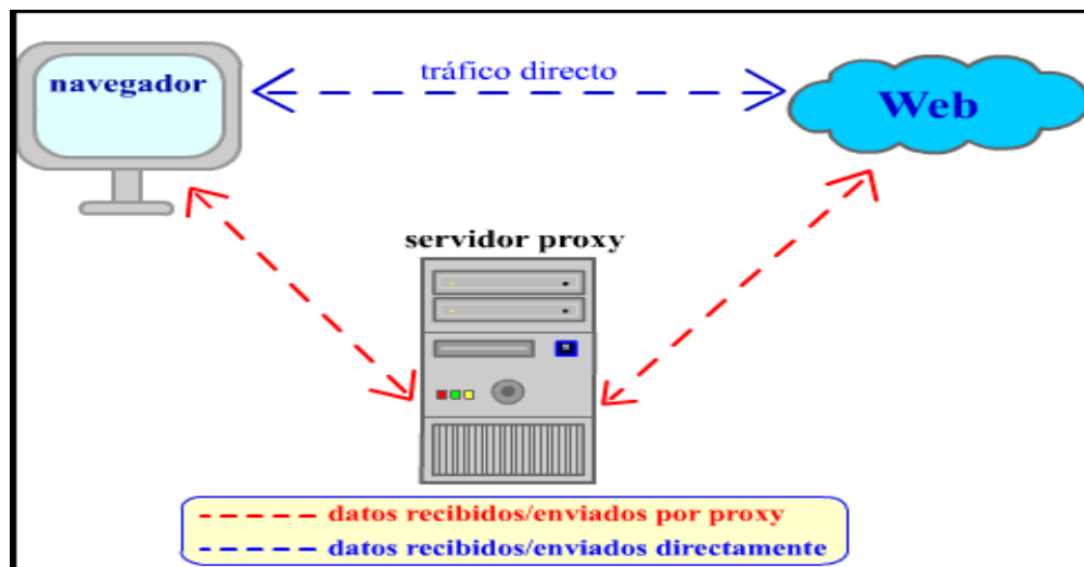
Figura 8.1 Funcionamiento de un servidor proxy. ( http://www.telypc.com , Parr 2)
