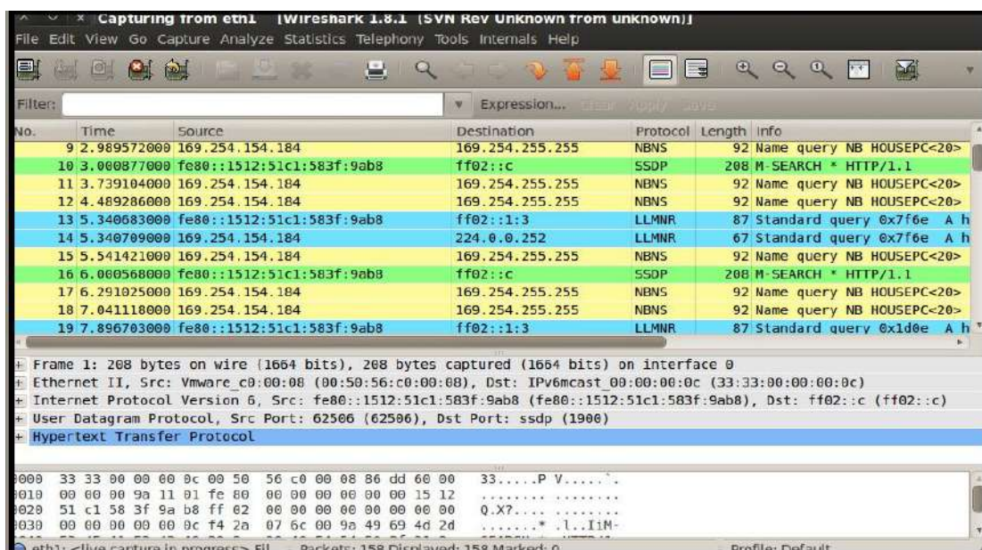
Figura 5.6 Visualización completa - Wireshark.
