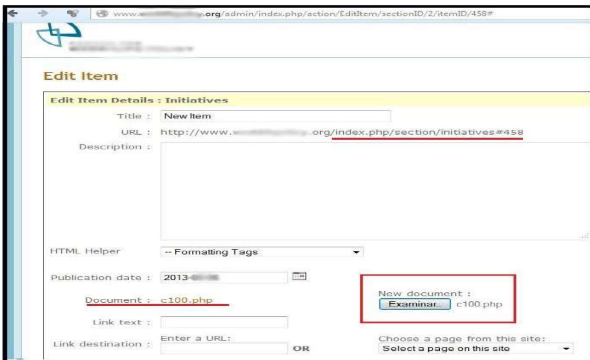
Figura 7.56 Subida de un WebShell en la Página Web – Web Analizada.
