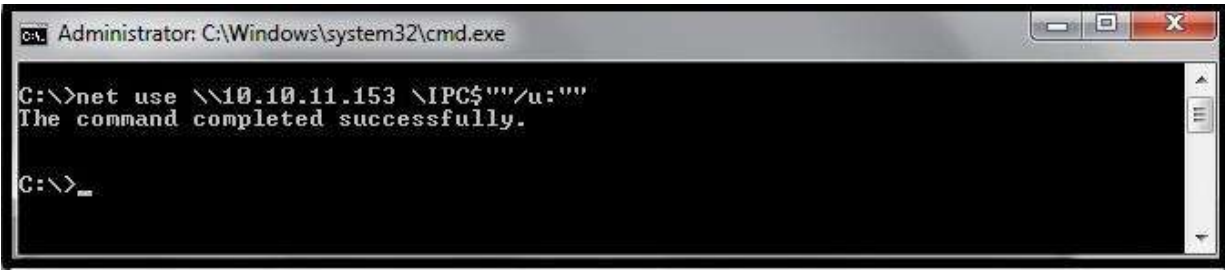
Figura 4.33 Ejecución del comando para iniciar una sesión nula – (D.O.S).
