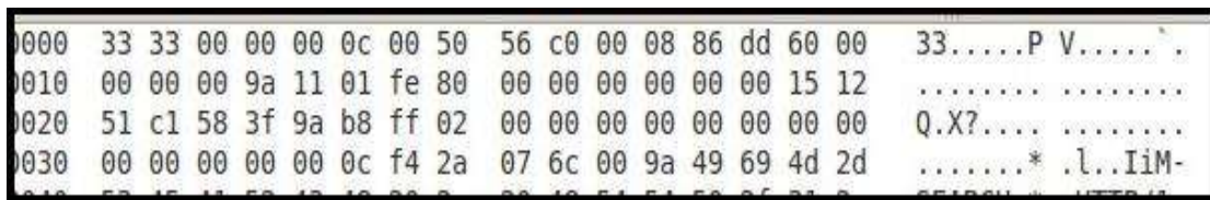
Figura 5.5 Panel de visualización por paquete en Bytes - Wireshark.
