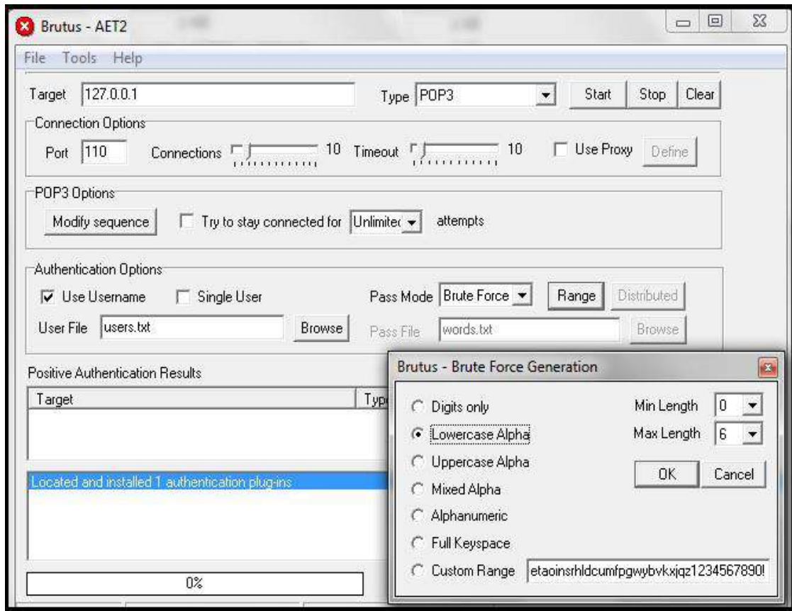
Figura 6.17 Aspecto visual de la herramienta – Brutus.
