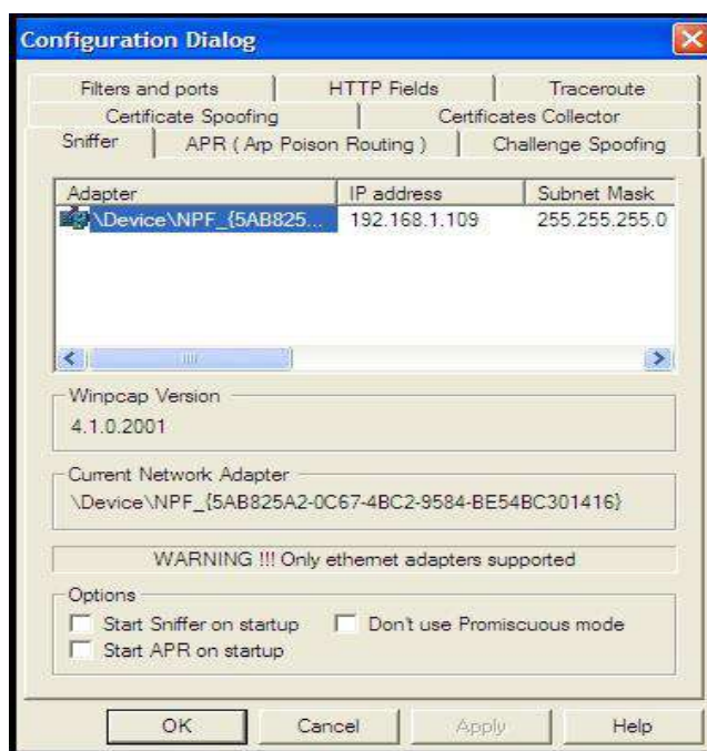
Figura 5.9 Configuración de la tarjeta de red – Cain y Abel.
