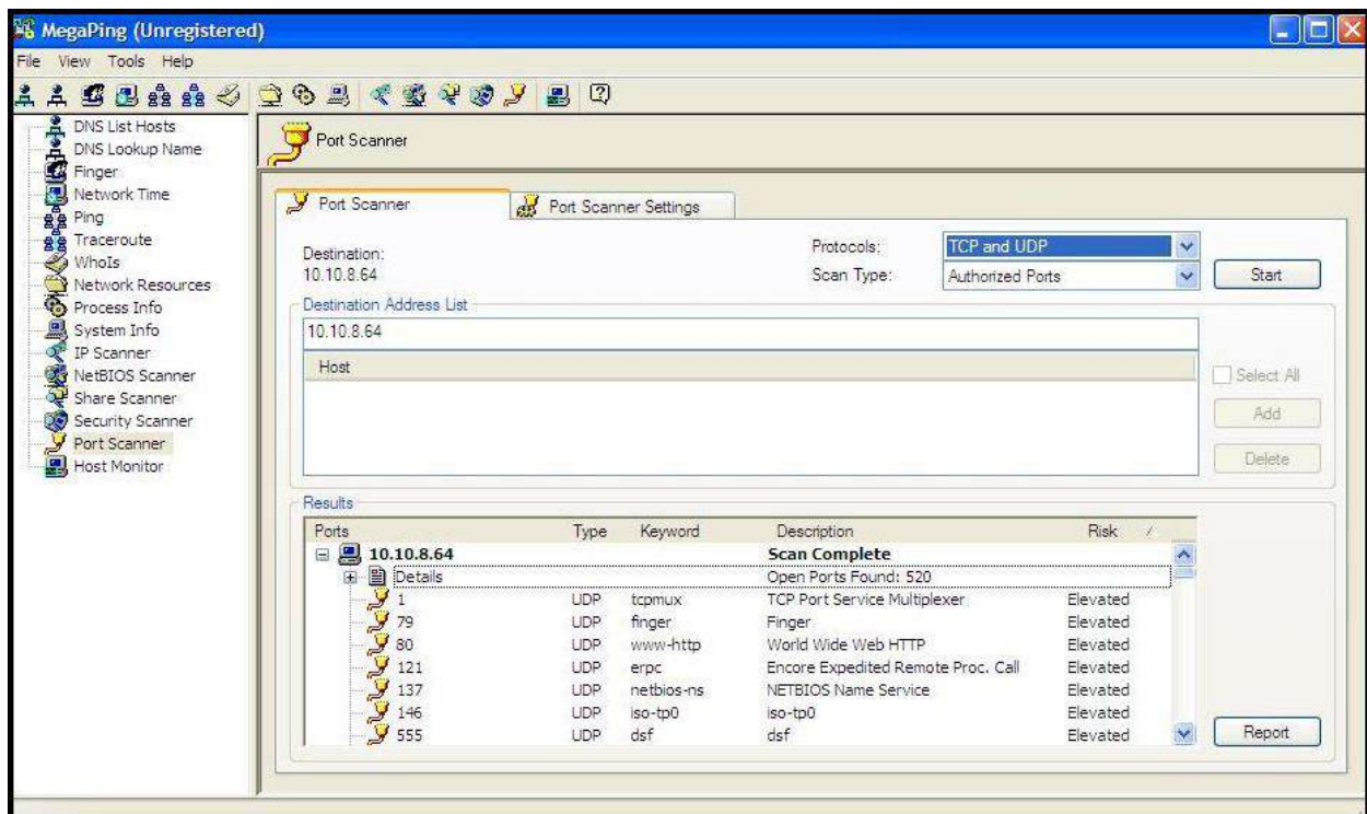
Figura 4.25 MegaPing - Análisis host vivos - Windows.
