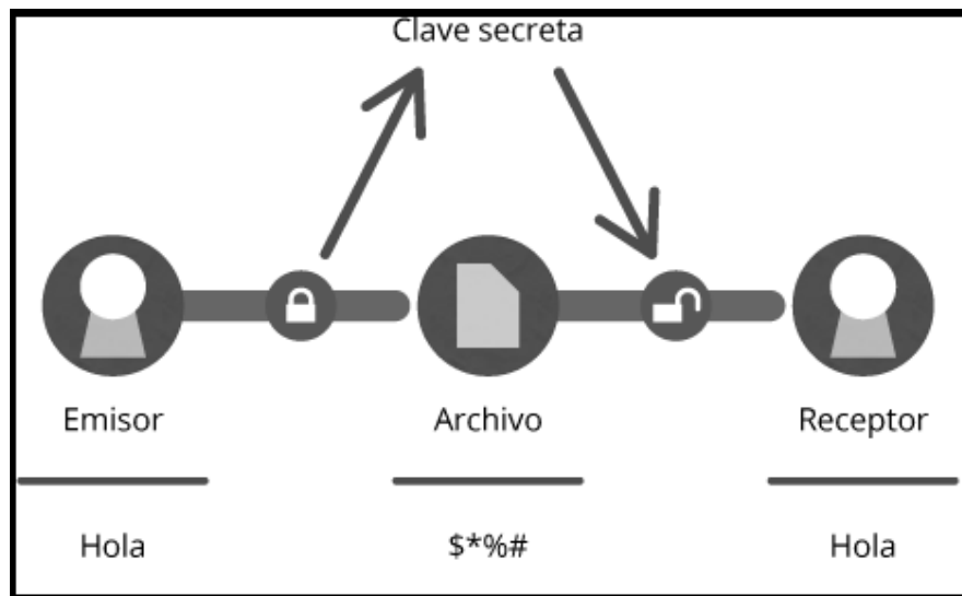
Figura 6.2 Funcionamiento de la Criptografía Simétrica. ( http://www.genbetadev.com )
