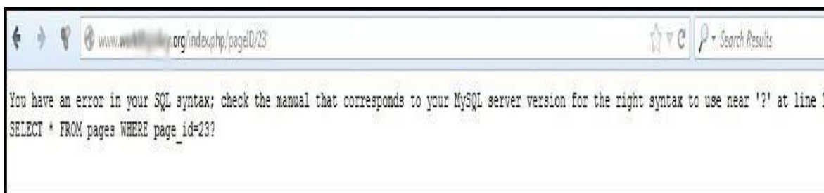
Figura 7.46 Inyección SQL para verificar vulnerabilidad – Web Analizada.
