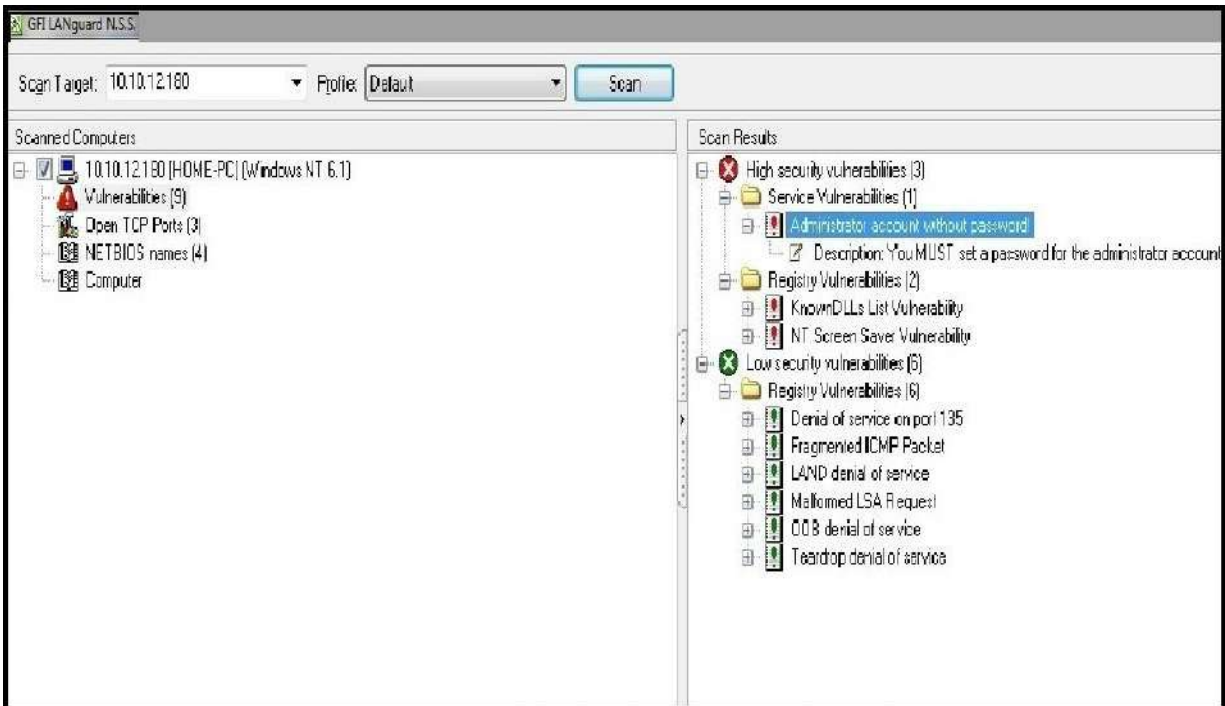
Figura 4.29 Escaneo de Vulnerabilidades a un Host en una LAN – Windows.
