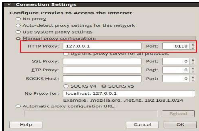
Figura 8.18 Configuración de Polipo en el browser – Firefox.
