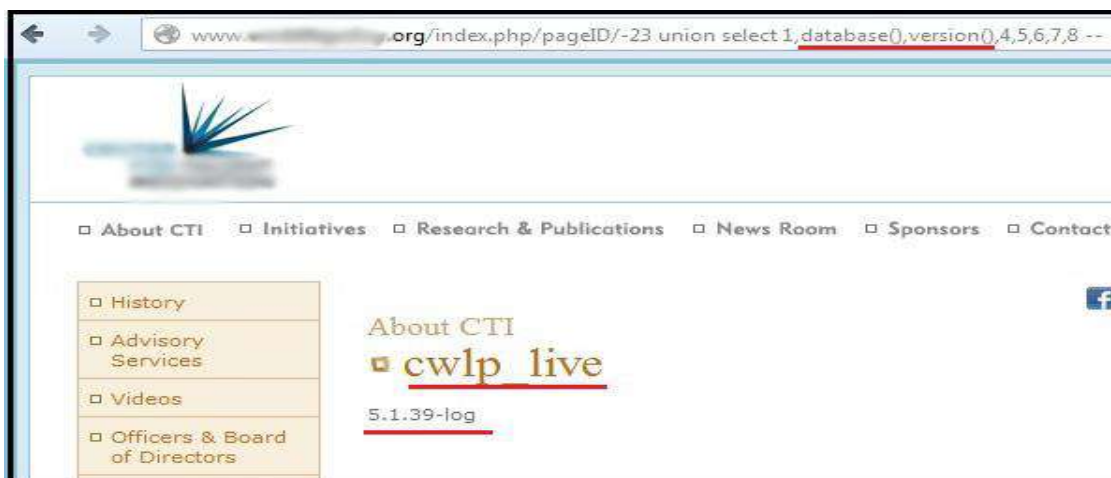
Figura 7.49 Consulta de Base de datos y versión del Gestor – Web Analizada.
