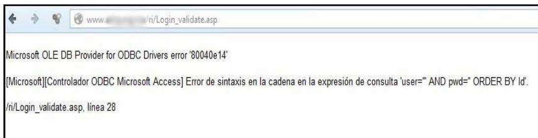
7.26 Verificación de error SQL Injection– Web Analizada.
