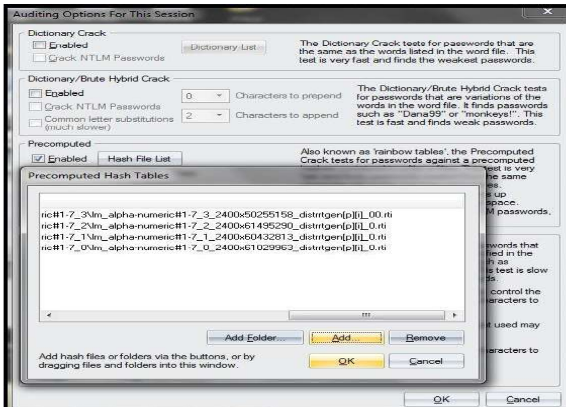
Figura 6.15 Selección del tipo de ataque – L0phtCrack
