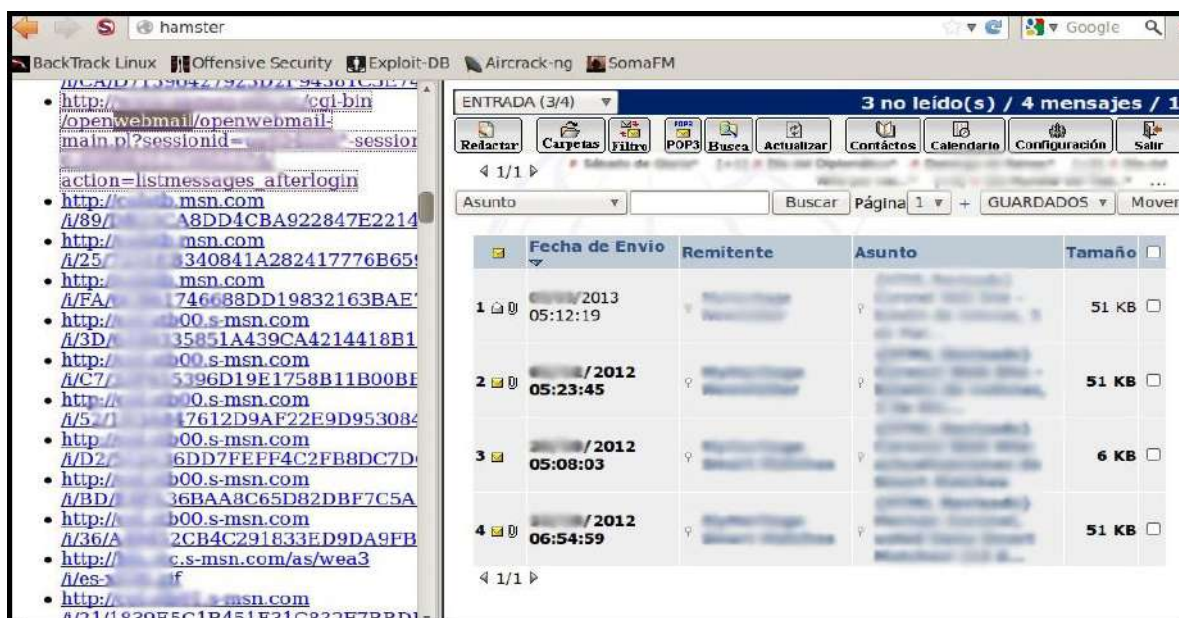
Figura 5.34 Captura de una Sesión de correo – Firefox.
