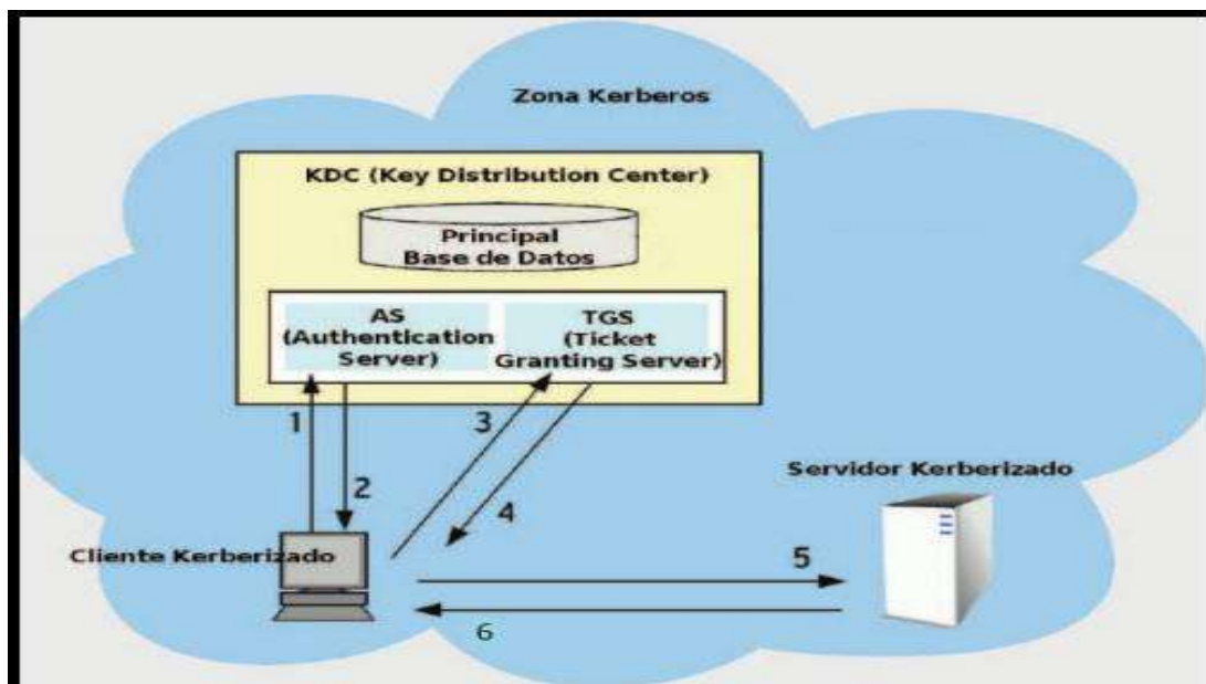
Figura 6.1 Autenticación con kerberos. ( http://www.webs.um.es/ , Parr 1)
