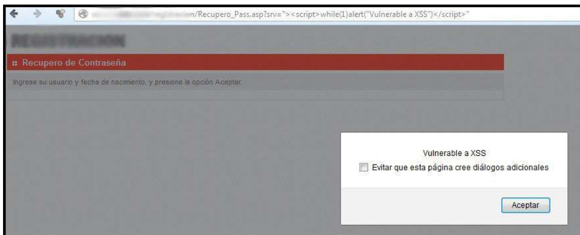
Figura 7.18 Comando para realizar XSS – Web Analizada.
