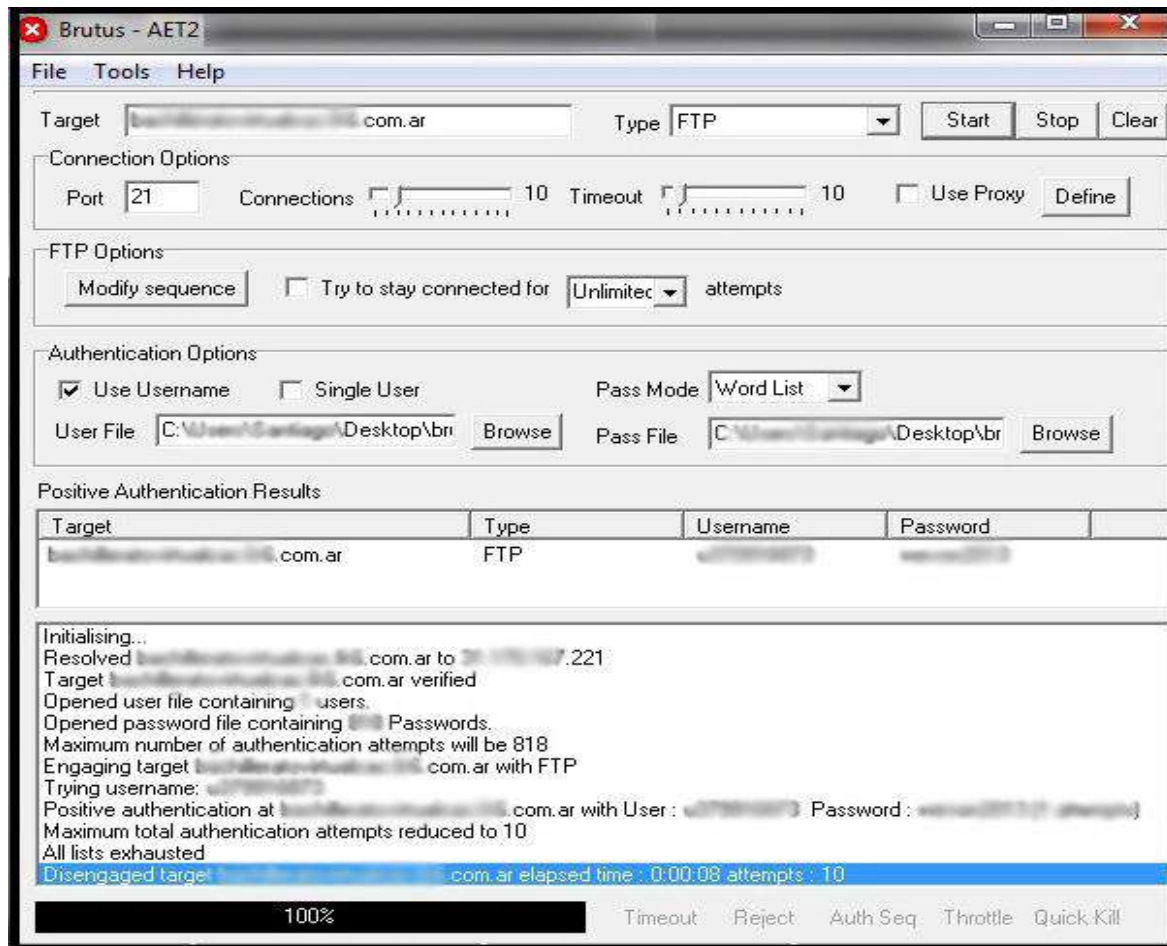
Figura 6.18 Aplicación de la herramienta Brutus – Windows.
