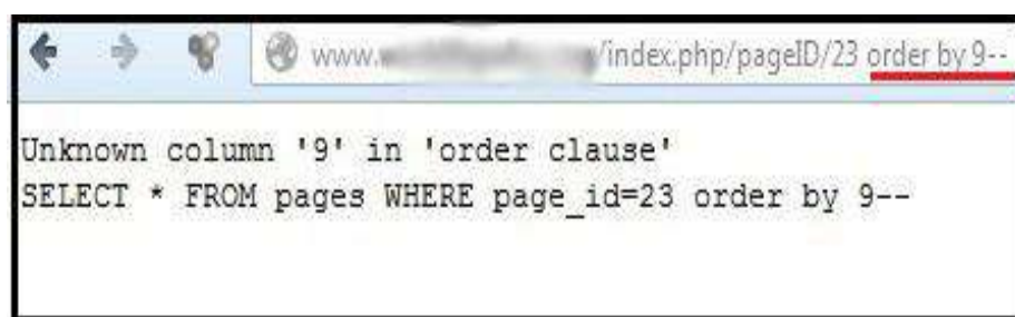
Figura 7.47 Obtención de campos habilitados – Web Analizada.
