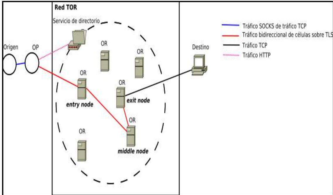
Figura 8.9 Funcionamiento de Tor ( http://es.wikipedia.org , Parr 5).
