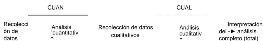
Figura 16.12. Esquema del diseño explicativo secuencial
