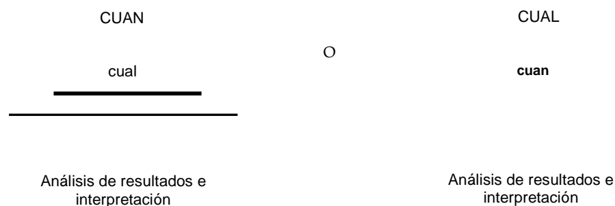
Figura 16.15. Diseños anidados concurrentes de modelo dominante. 18
