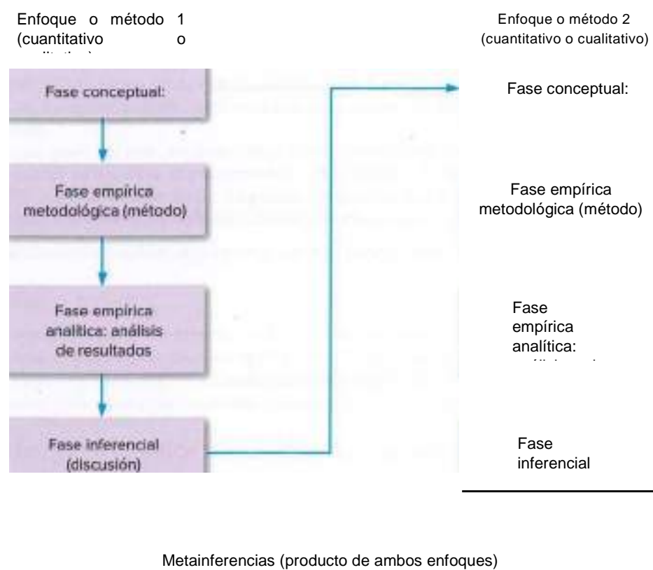
Figura 16.7. Procesos de los diseños mixtos secuenciales.
